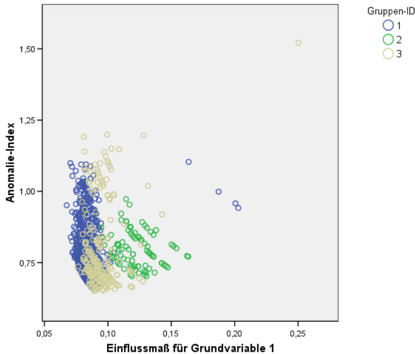
Abbildung 9-17 Streudiagramm des Anomalie-Index über das Einflussmaß der ersten Grundvariablen
