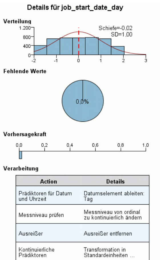
Abbildung 8-10 Felddetails für job_start_date_day
