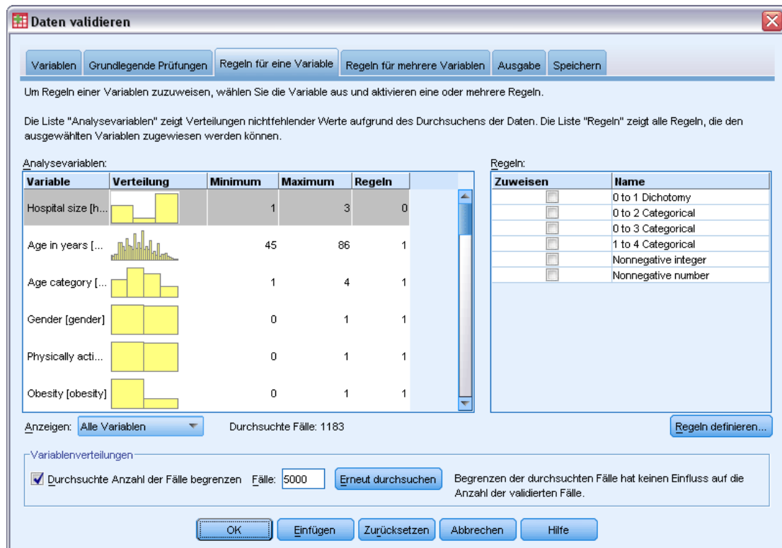
Abbildung 3-4 Dialogfeld "Daten validieren," Registerkarte "Regeln für eine Variable"
