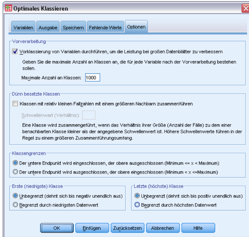
Abbildung 6-5 Dialogfeld “Optimales Binning”; Registerkarte “Optionen”
