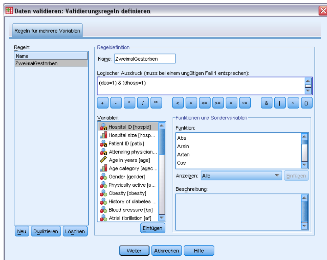
Abbildung 7-24 Dialogfeld "Validierungsregeln definieren", Registerkarte "Regeln für mehrere Variablen"
