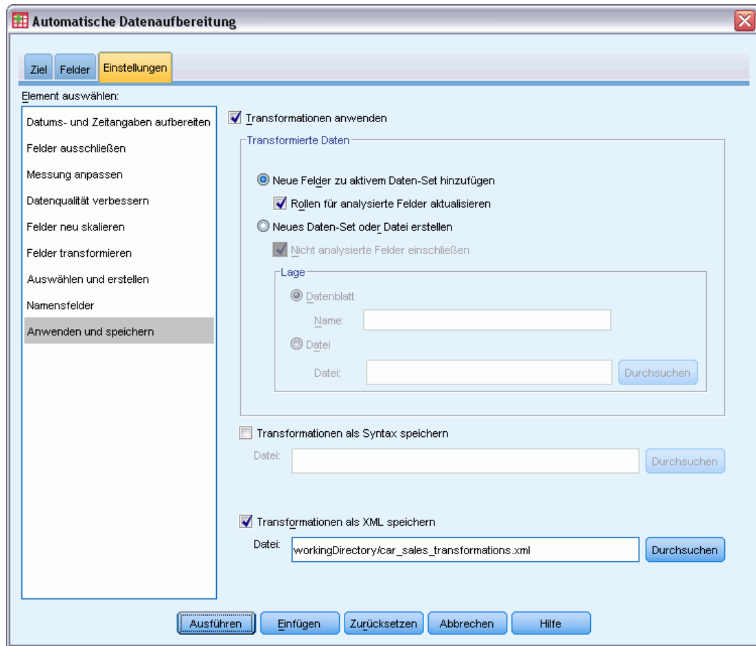
Abbildung 8-13 Einstellungen "Anwenden und speichern"
