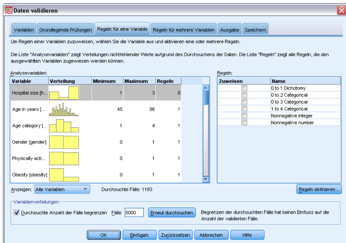
Abbildung 7-10 Dialogfeld "Daten validieren," Registerkarte "Regeln für eine Variable"
