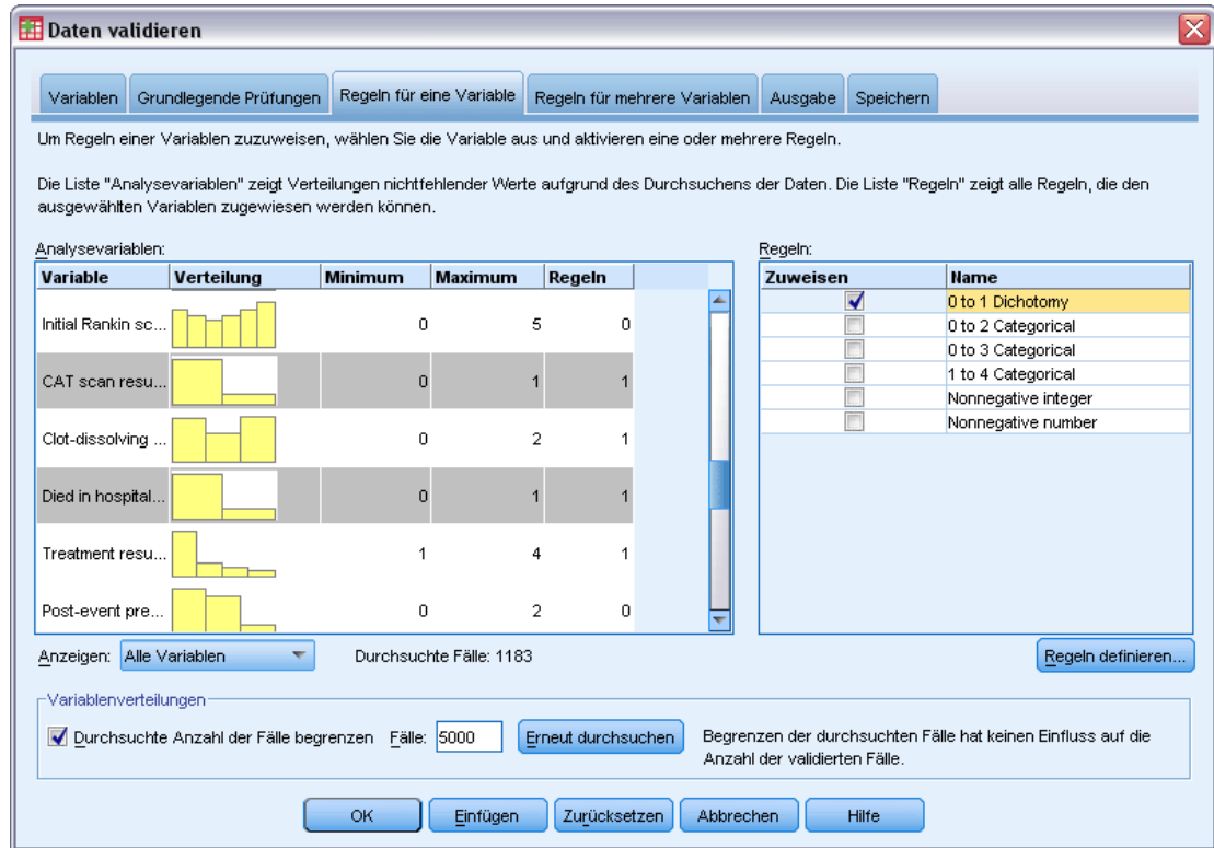
Abbildung 7-11 Dialogfeld "Daten validieren," Registerkarte "Regeln für eine Variable"
