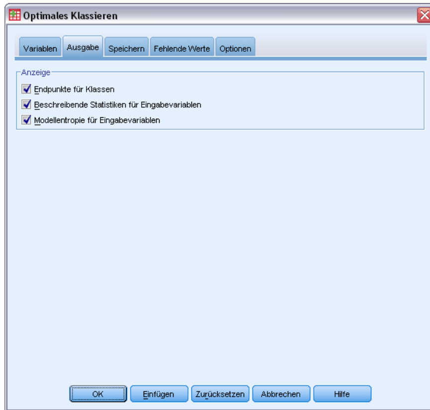
Abbildung 10-2 Dialogfeld "Optimales Klassieren," Registerkarte "Ausgabe"
