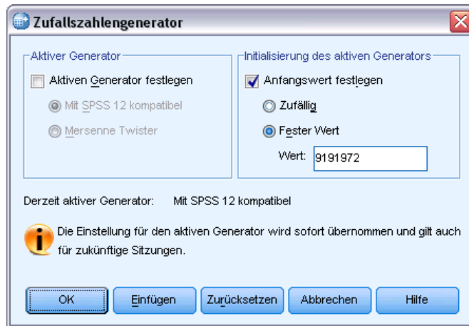
Abbildung 4-23 Dialogfeld "Zufallszahlengenerator"
