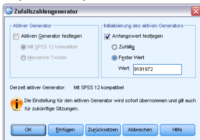
Abbildung 5-1 Dialogfeld ‘‘Zufallszahlengenerator’’
