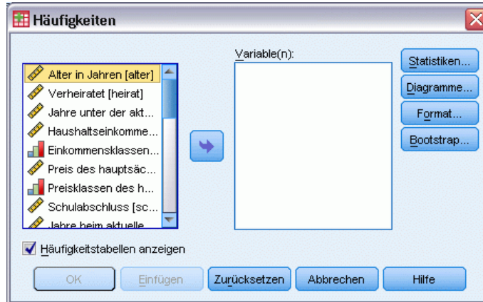
Abbildung 1-5 Dialogfeld “Häufigkeiten”
