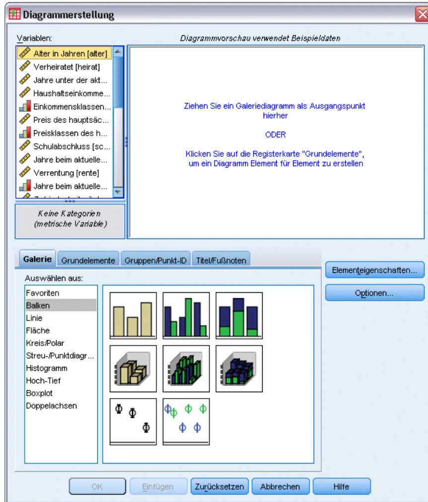
Abbildung 6-1 Dialogfeld “Diagrammerstellung”
