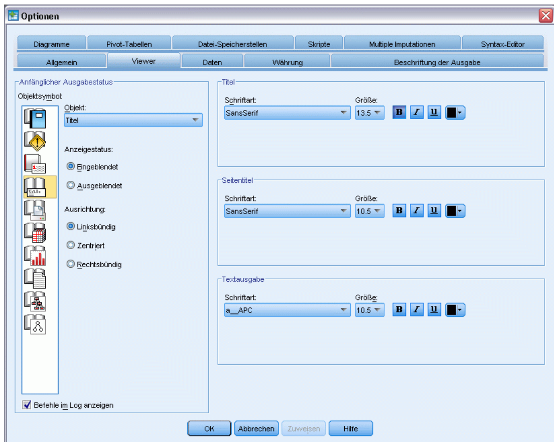
Abbildung 7-18 Optionen: Viewer
