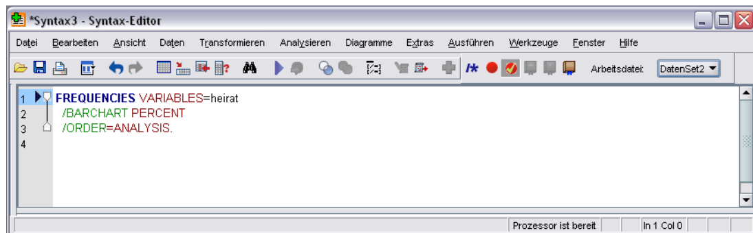
Abbildung 8-2 Häufigkeitssyntax
