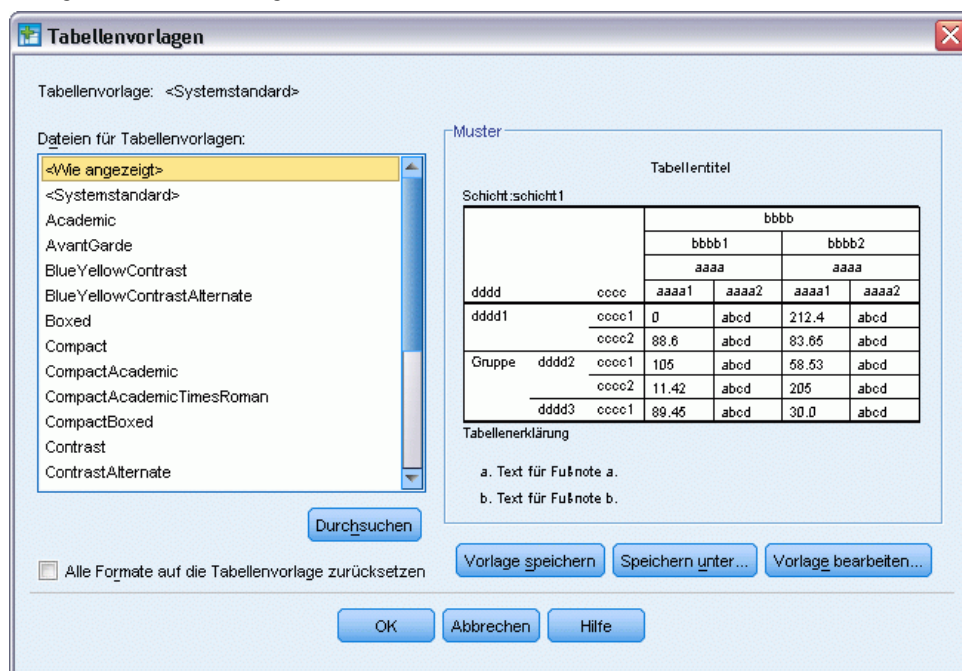
Abbildung 7-13 Dialogfeld “Tabellenvorlagen”
