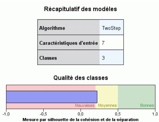
Figure 24-5 Vue récapitulative du modèle du panneau principal
