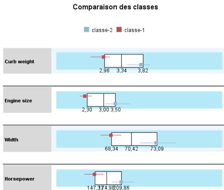
Figure 24-11 Vue de comparaison des classes dans le panneau des liens
