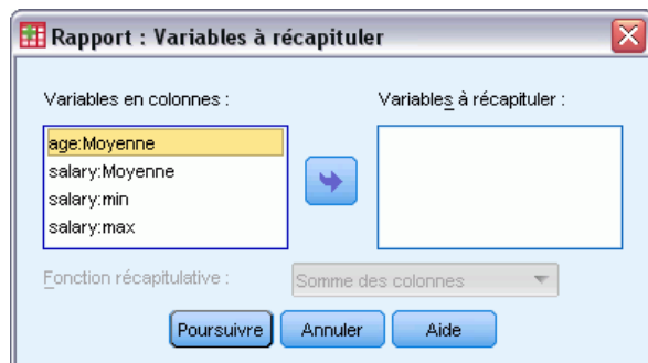
Figure 29-10 Boîte de dialogue Tableau de bord : Colonnes
