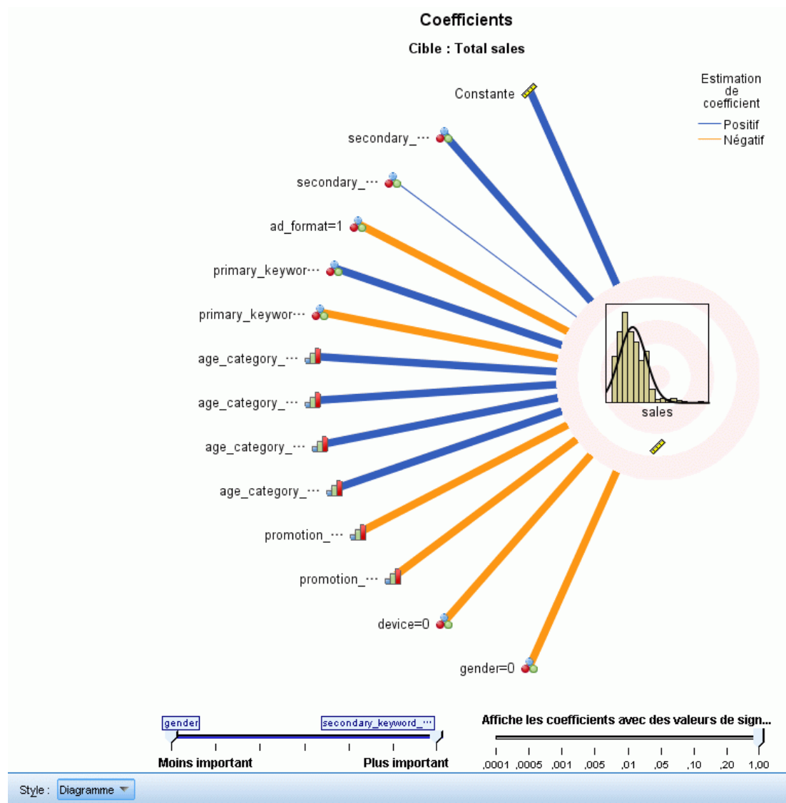
Figure 15-15 Vue Coefficients, style de diagramme
