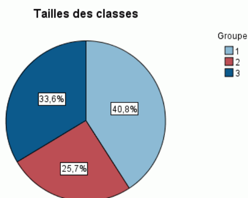
Figure 24-9 Vue de la taille des classes dans le panneau des liens
