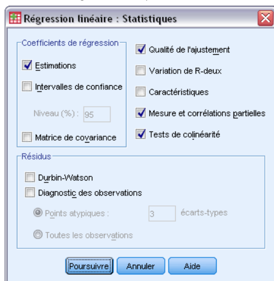
Figure 16-5 Boîte de dialogue Statistiques
