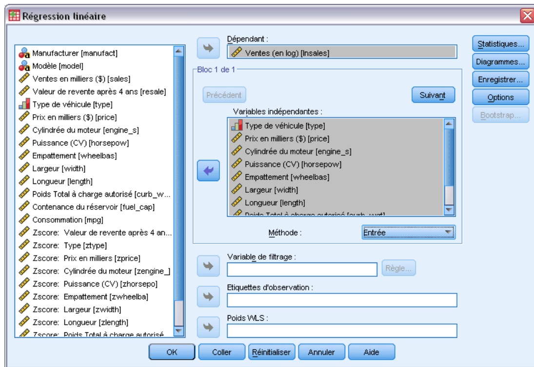
Figure 16-1 Boîte de dialogue Régression linéaire
