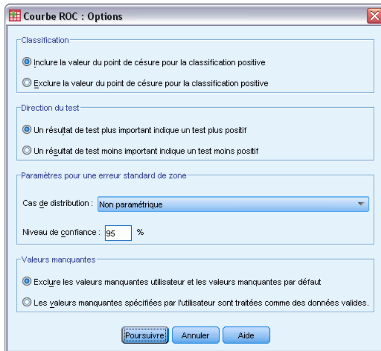
Figure 33-2 Boîte de dialogue Courbe ROC : Options
