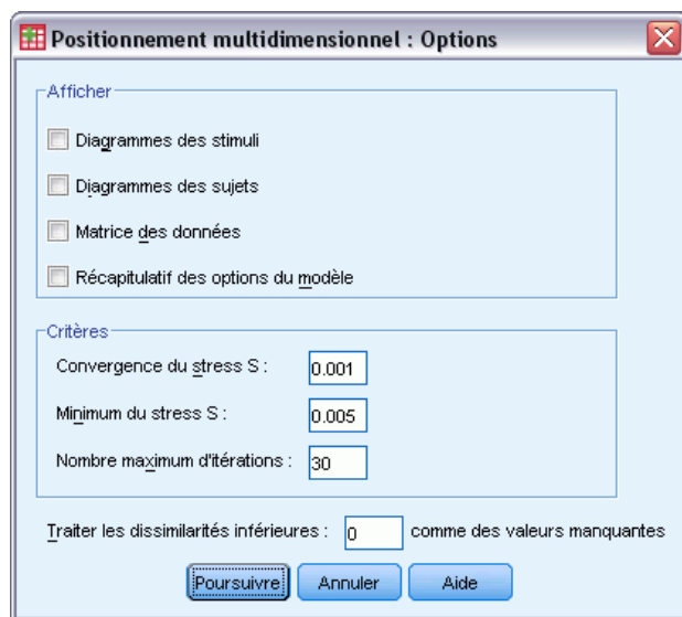
Figure 31-5 Boîte de dialogue Positionnement multidimensionnel : Options
