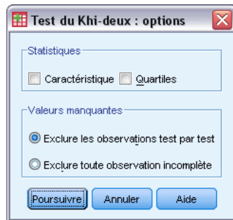
Figure 27-50 Boîte de dialogue Test du Khi-deux : Options
