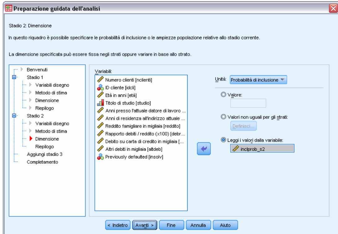
Figura 14-13 Preparazione guidata dell'analisi - Passo Dimensione (stadio 2)
