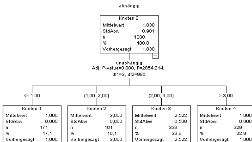
Abbildung 3-3 Baum, bei dem beide Variablen als metrische Variablen behandelt werden
