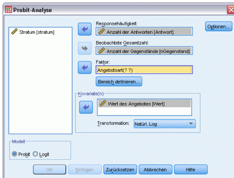
Abbildung 4-1 Dialogfeld "Probit-Analyse"
