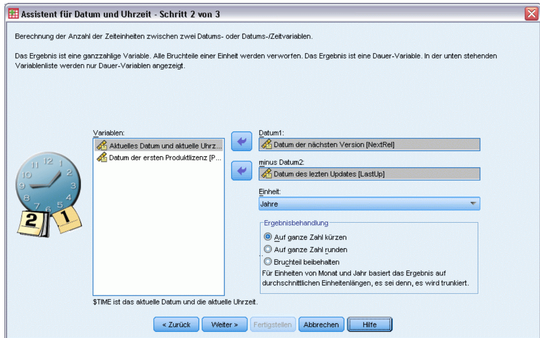
Abbildung 8-24 Subtrahieren von Datumswerten, Schritt 2
