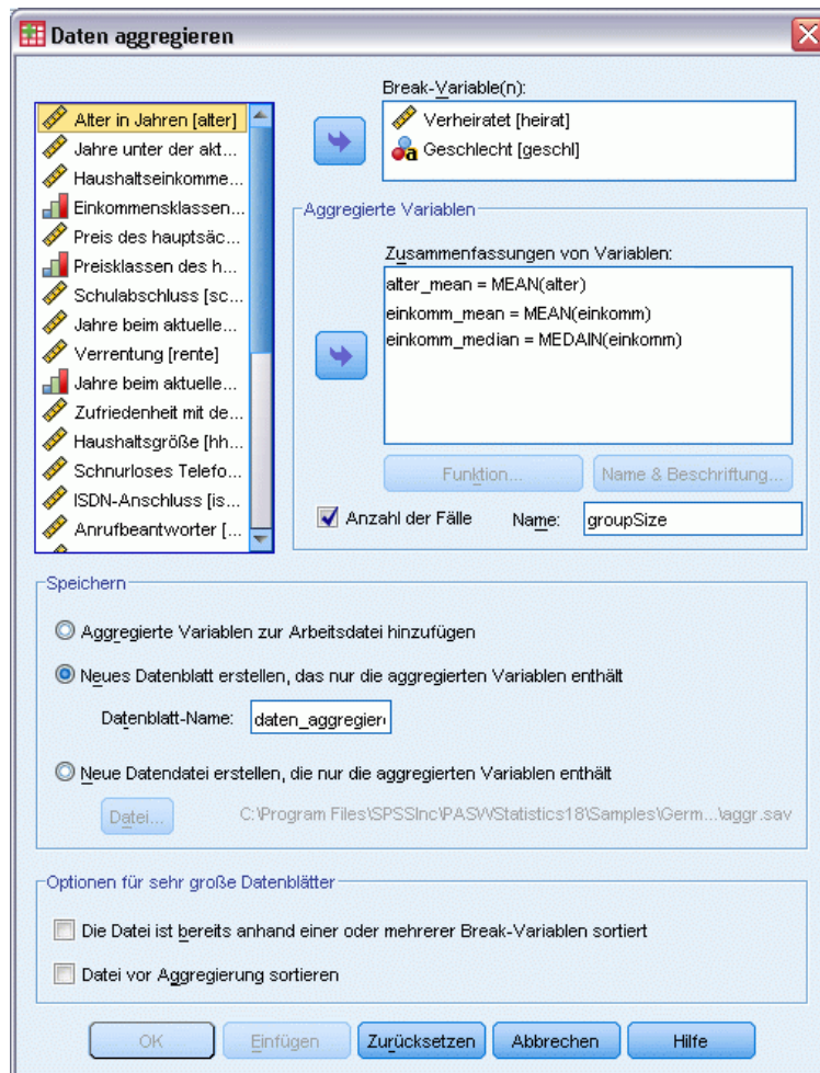
Abbildung 9-5 Dialogfeld "Daten aggregieren"
