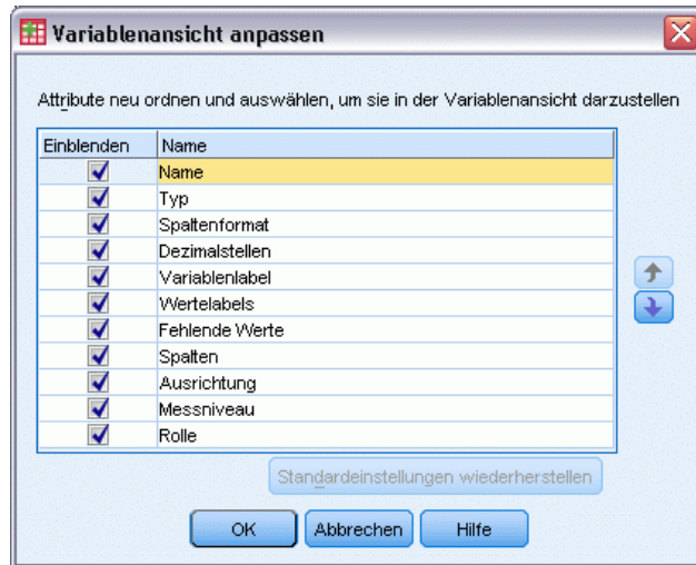
Abbildung 5-8 Variablenansicht anpassen
