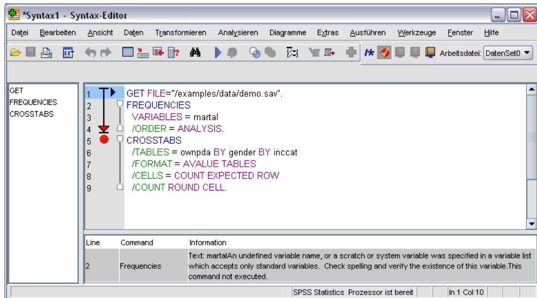
Abbildung 13-3 Syntax-Editor
