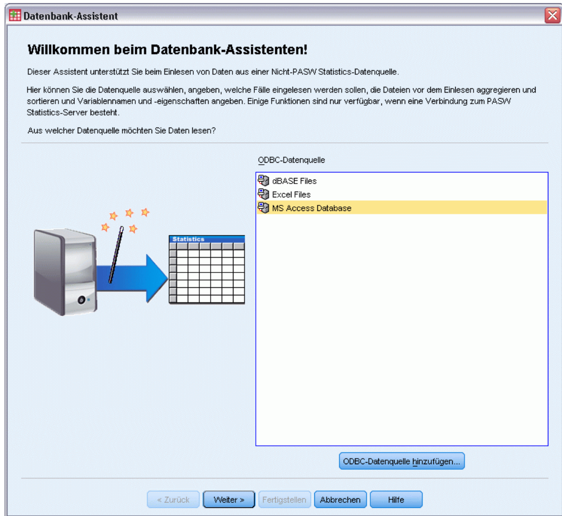
Abbildung 3-1 Datenbank-Assistent
