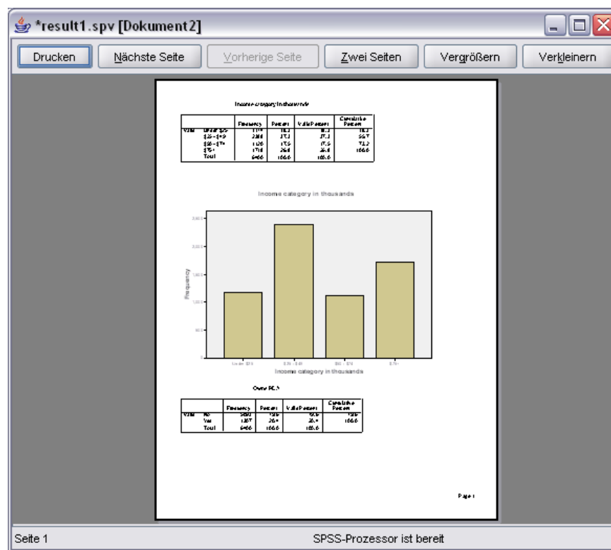
Abbildung 10-7 Seitenansicht
