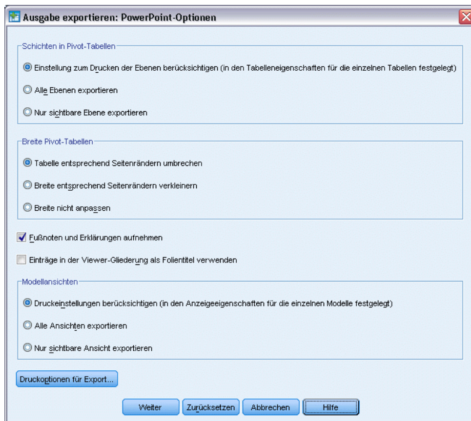
Abbildung 10-3 Dialogfeld "Powerpoint-Exportoptionen"
