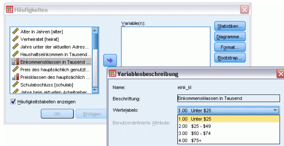
Abbildung 1-3 Variablenbeschreibung
