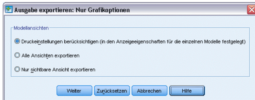
Abbildung 10-6 Nur Grafikoptionen
