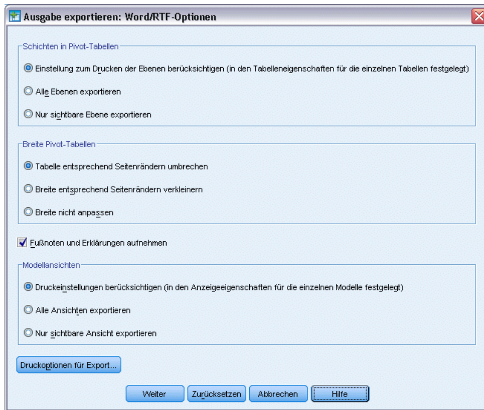
Abbildung 10-2 Optionen zum Exportieren von Word-Ausgaben
