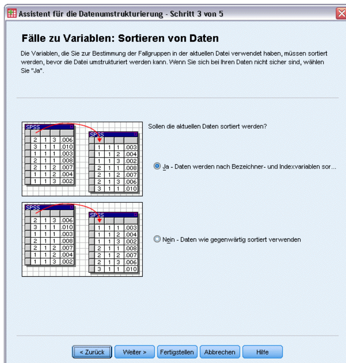
Abbildung 9-31 Assistent für die Datenumstrukturierung: Sortieren von Daten, Schritt 3
