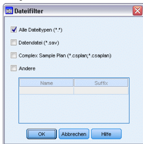
Abbildung 19-4 Dialogfeld "Dateifilter"
