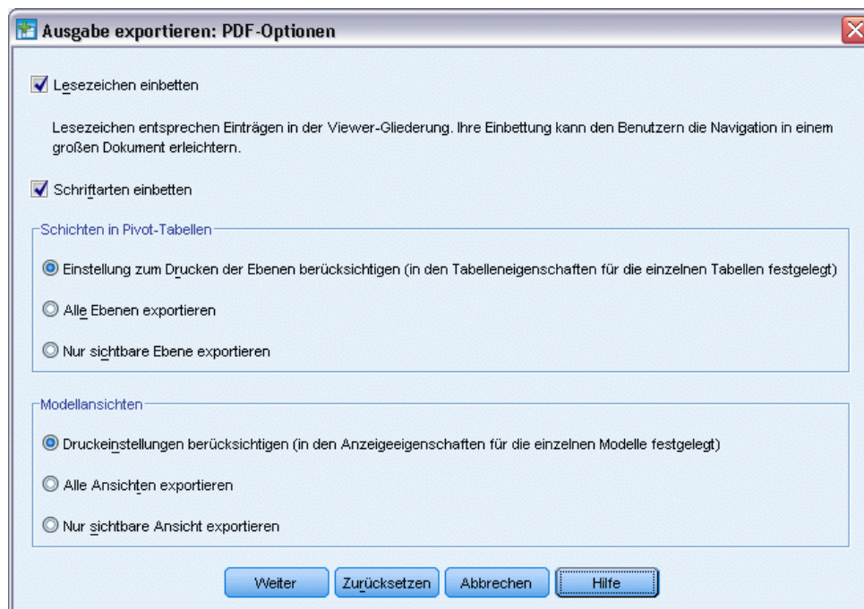
Abbildung 10-4 Dialogfeld "PDF-Optionen"
