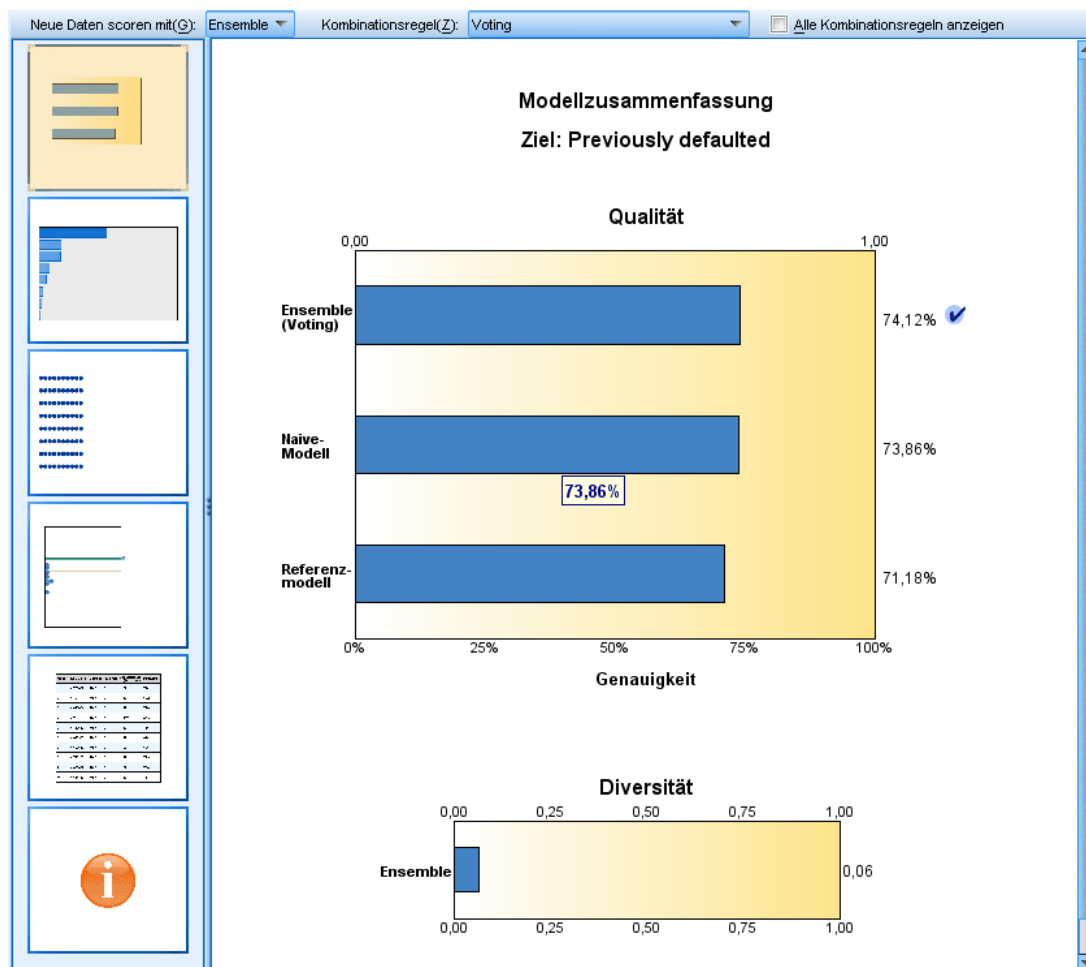
Abbildung 12-4 Ansicht "Modellzusammenfassung"
