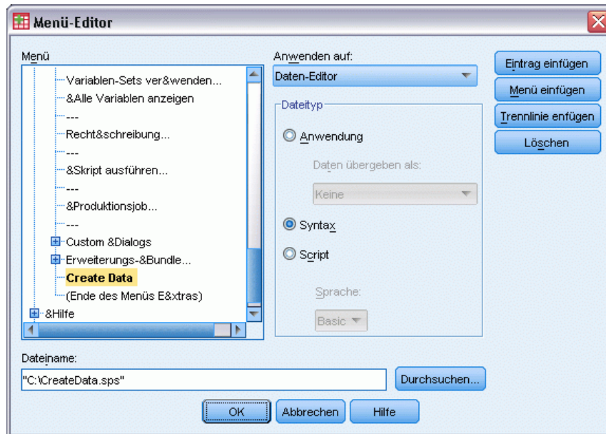
Abbildung 18-1 Dialogfeld "Menü-Editor"
