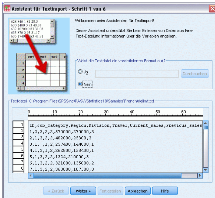
Abbildung 3-13 Text-Assistent: Schritt 1
