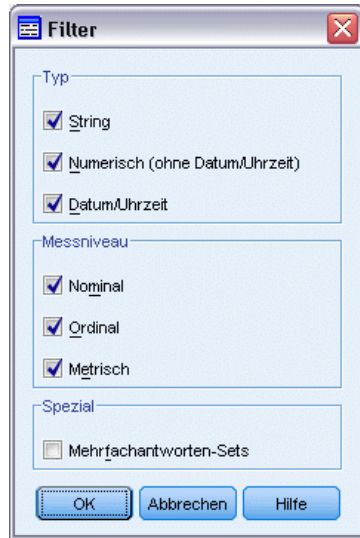
Abbildung 19-3 Dialogfeld "Filter"
