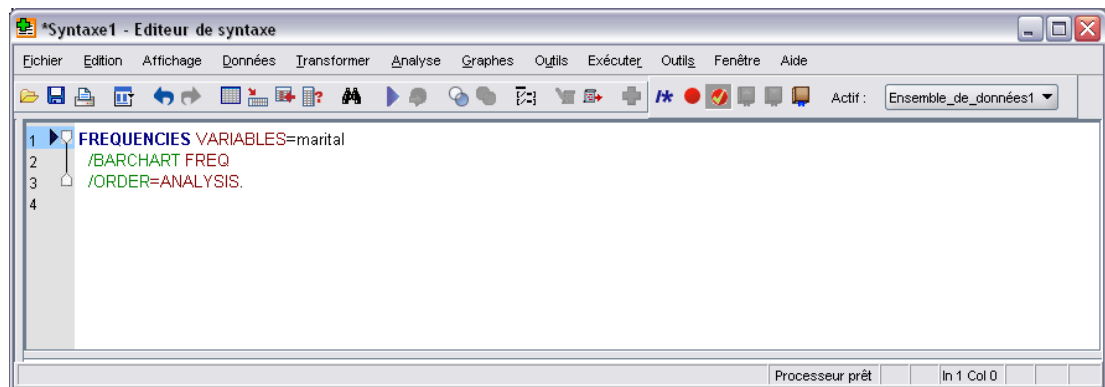
Figure 8-2 Syntaxe d'effectifs
