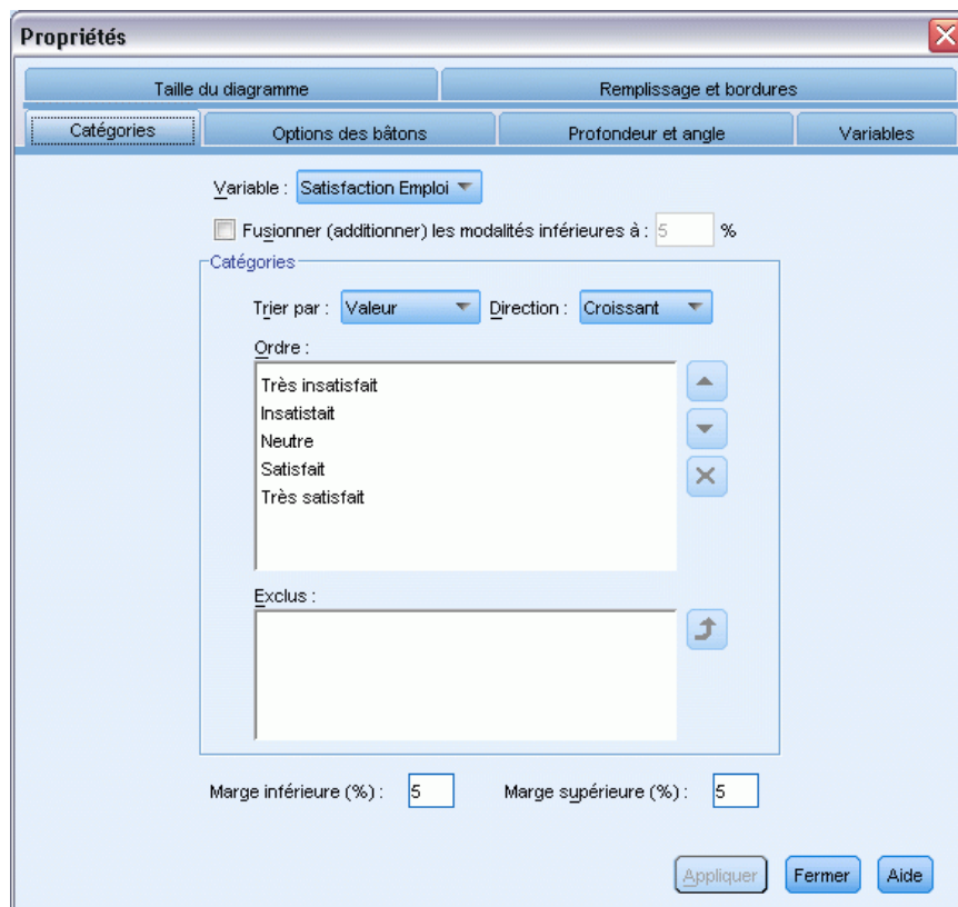
Figure 6-8 Fenêtre Propriétés
