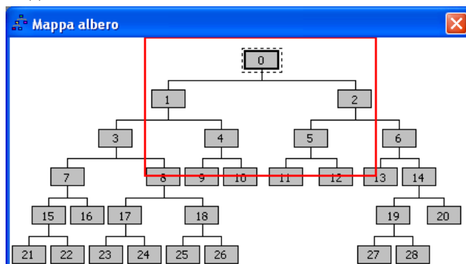
Figura 5-5 Mappa dell'albero
