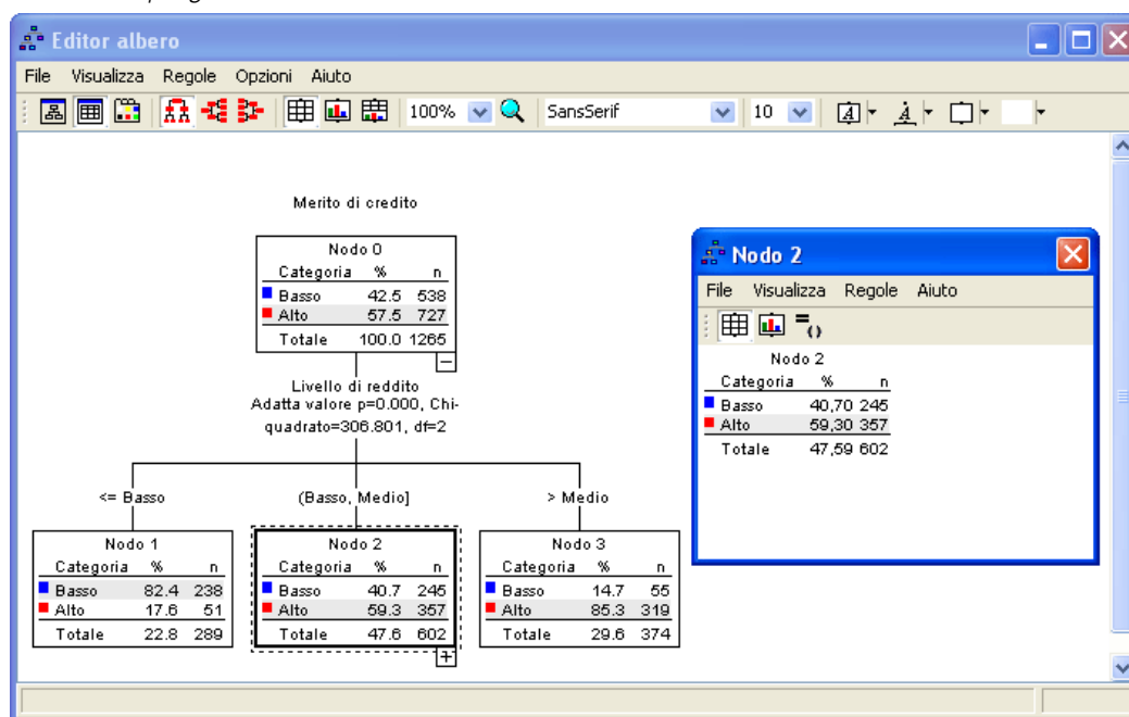
Figura 2-4 Finestra Riepilogo
