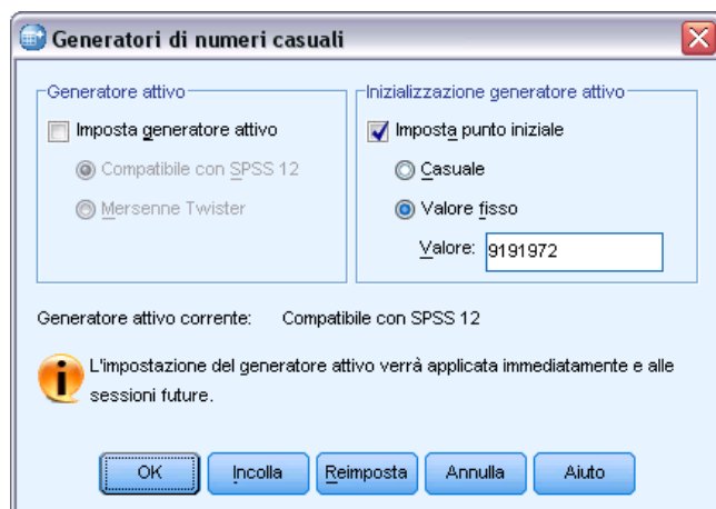
Figura 4-23 Finestra di dialogo Generatori di numeri casuali
