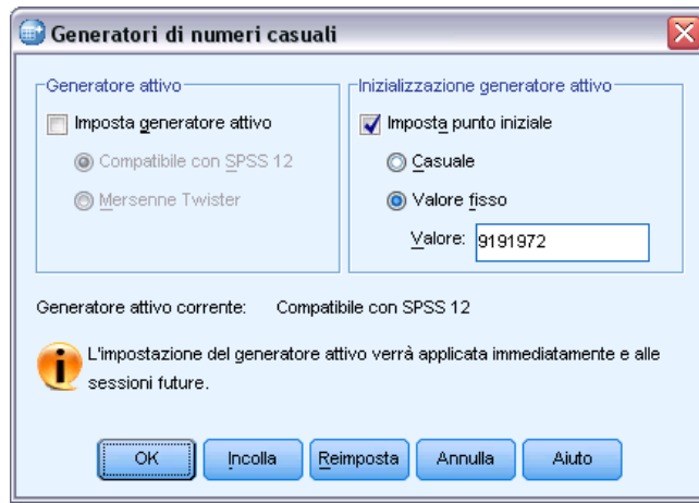
Figura 4-1 Finestra di dialogo Generatori di numeri casuali
