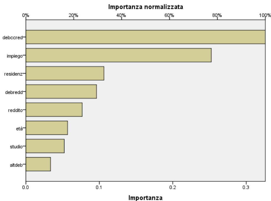
Figura 4-22 Grafico dell'importanza delle variabili indipendenti
