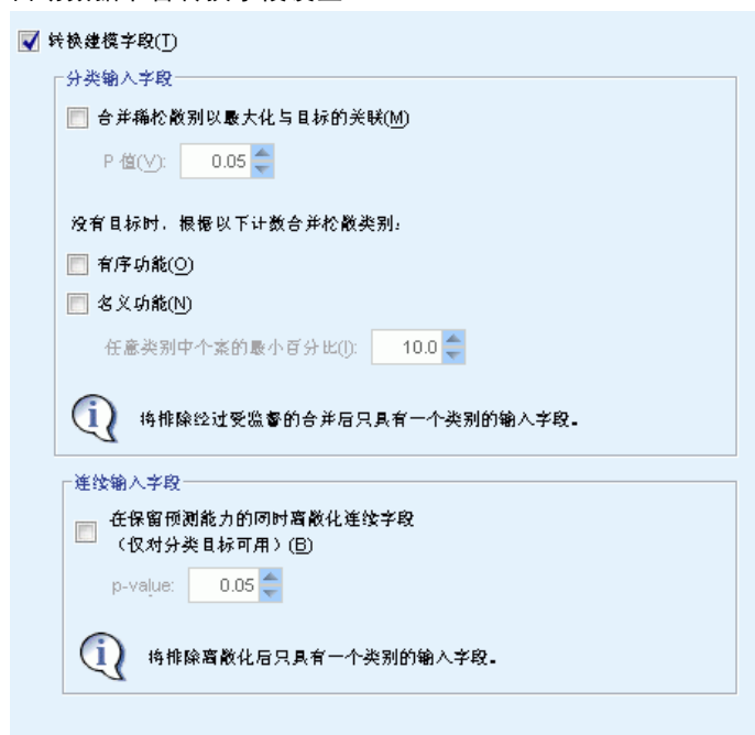
图片 4-8 自动数据准备转换字段设置
