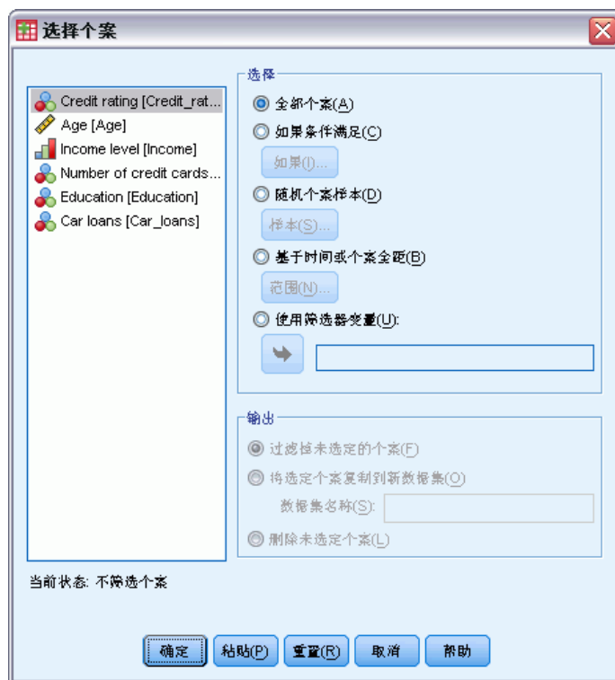
图片 4-21 “选择个案”对话框
