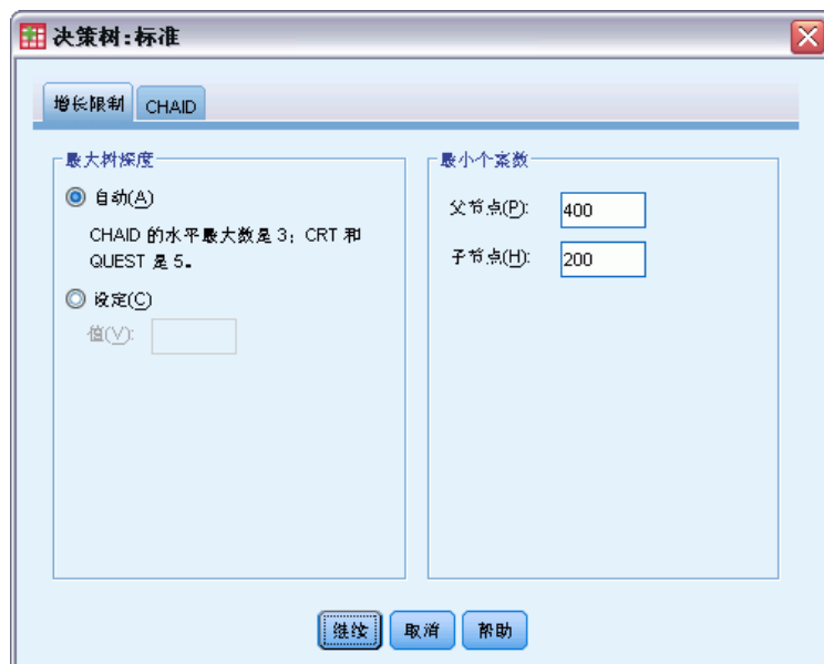
图片 6-3 “条件”对话框，“增长限制”选项卡
