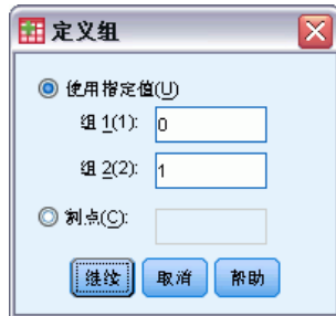
图片 9-2 数值变量的“定义组”对话框
