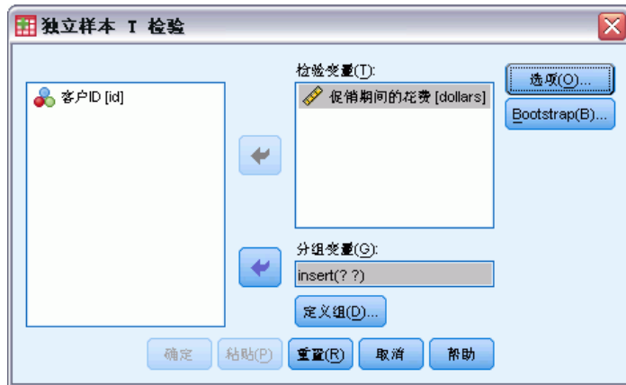
图片 9-1 “独立样本 T 检验”对话框
