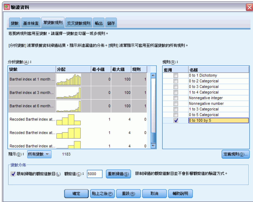
圖表 7-23 「驗證資料」對話方塊，「單一變數規則」索引標籤（已定義 0 到 100 類別，每 5 個定義為一類別）
