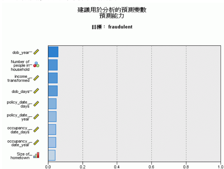
圖表 8-7 分析索引標籤，最佳化準確度時的預測能力
