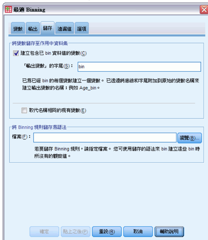
圖表 6-3 「最適 Binning」對話方塊，「儲存」索引標籤
