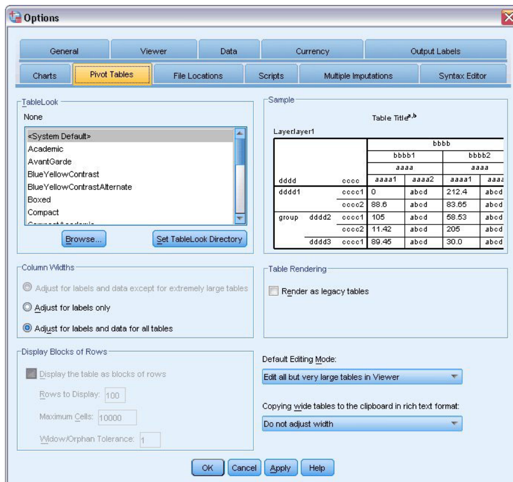
Figure 49. Boîte de dialogue Options
