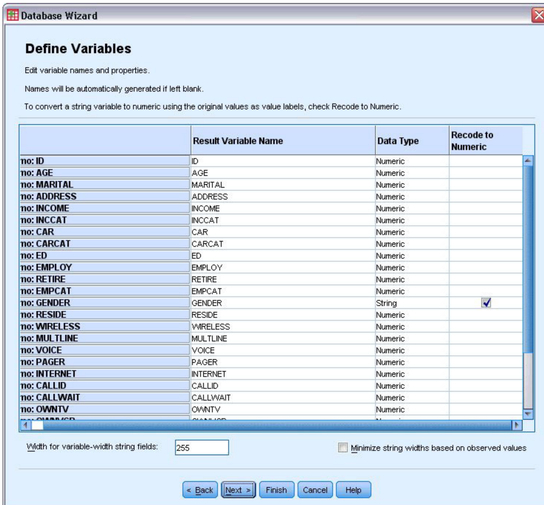
Figure 14. Etape de définition des variables
