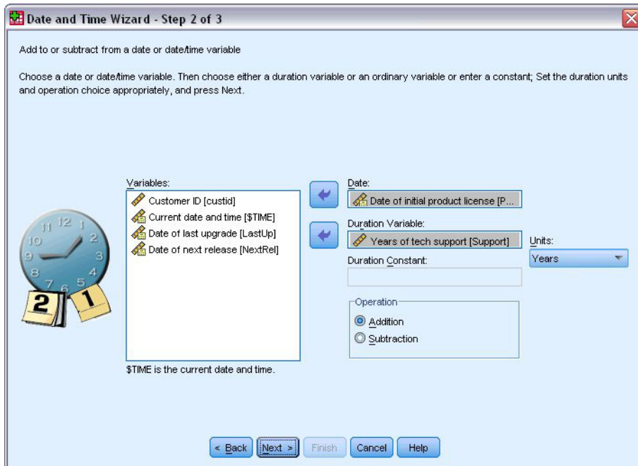
Figure 76. Ajout d'une durée à une date : Etape 2
