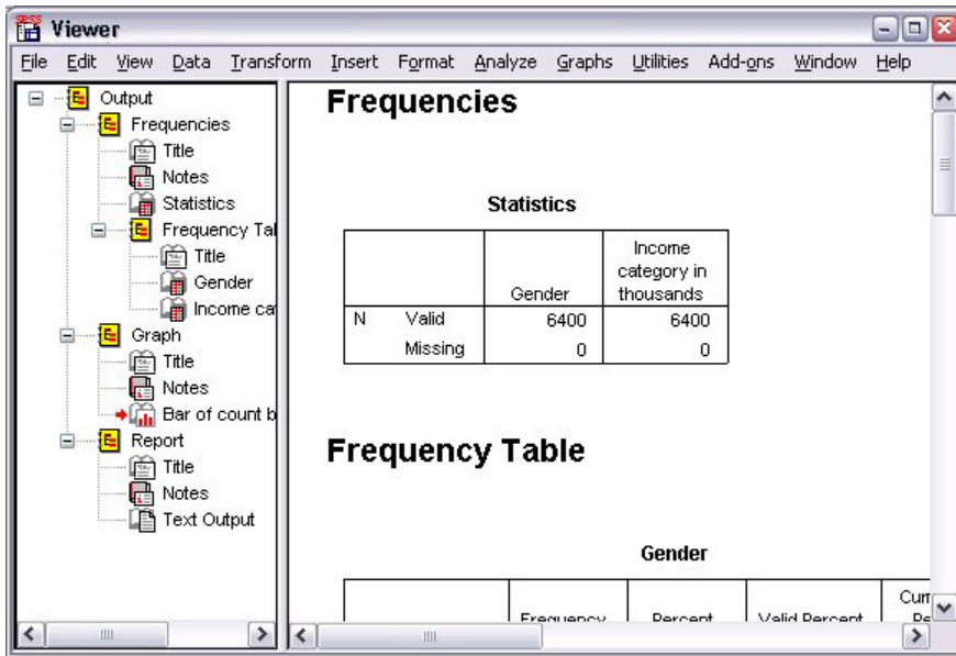
Figure 54. Visualiseur
