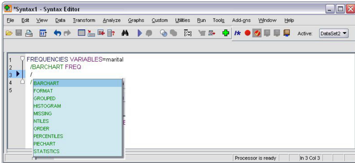
Figure 69. Contrôle de saisie semi-automatique affichant les sous-commandes
