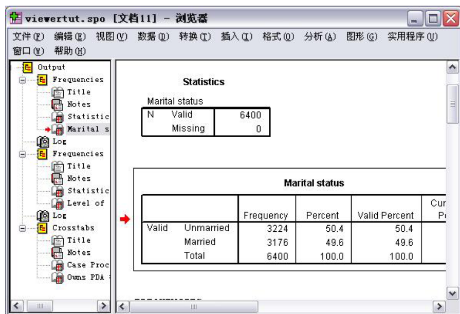
图 35. 查看器(V)
