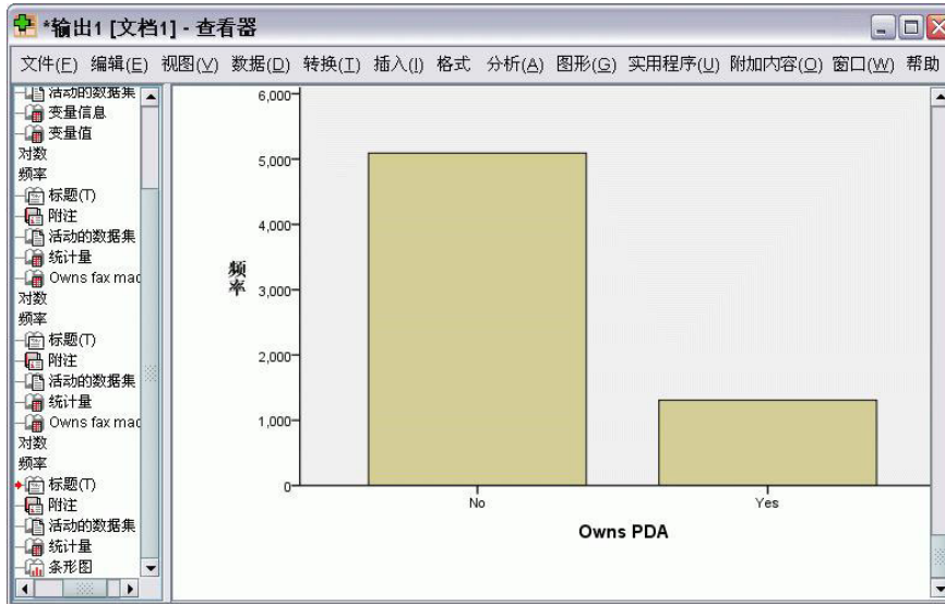
图 27. 条形图
