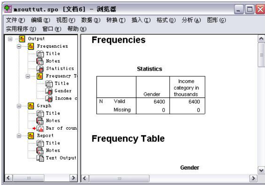
图 54. 查看器(V)
