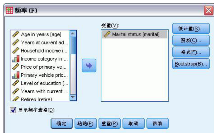
图 67. “频率”对话框
