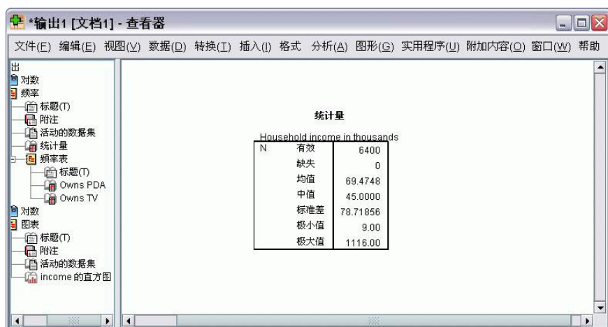
图 28. “频率统计”表
