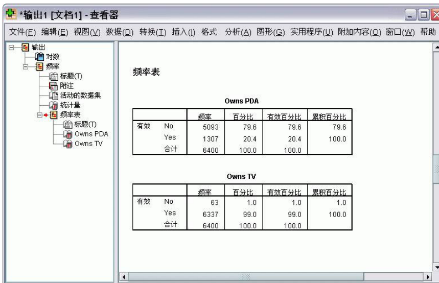
图 25. 频率表
