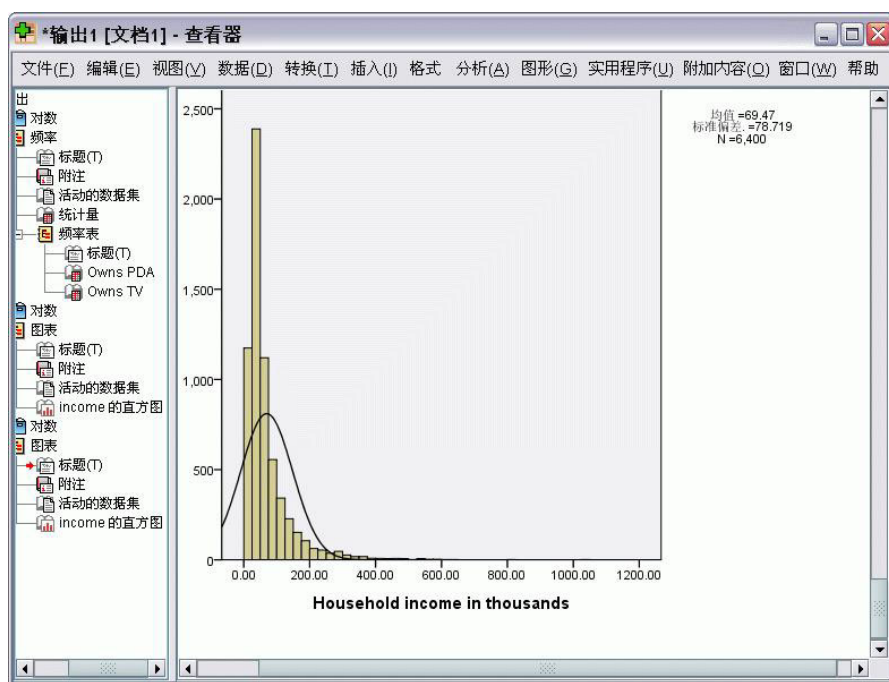
图 29. 直方图
