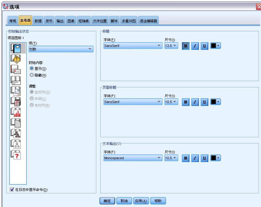
图 50. 查看器选项
