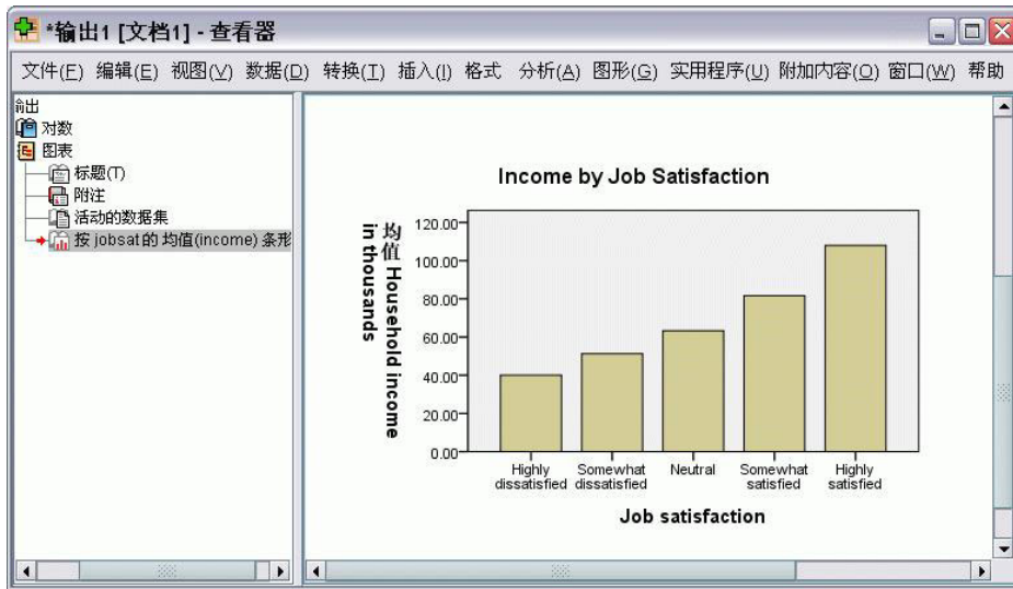
图 34. 条形图
