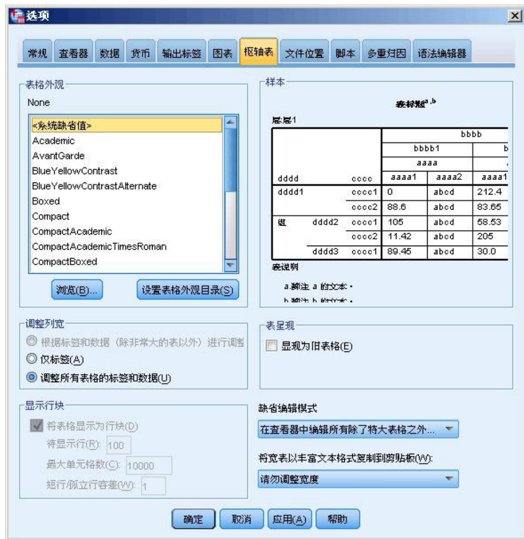
图 49. “选项”对话框
