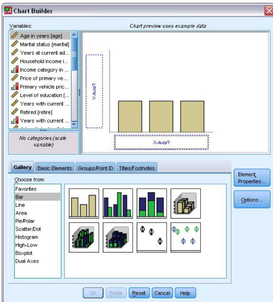
Abbildung 31. Balkendiagramm im Erstellungsbereich für die Diagrammerstellung
