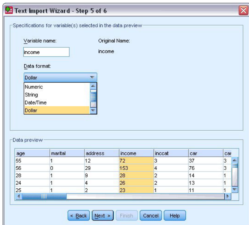
Figura 16. Modificare il tipo di dati
