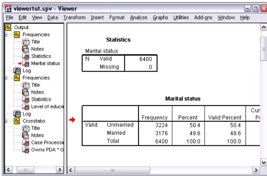
그림 35. 뷰어
