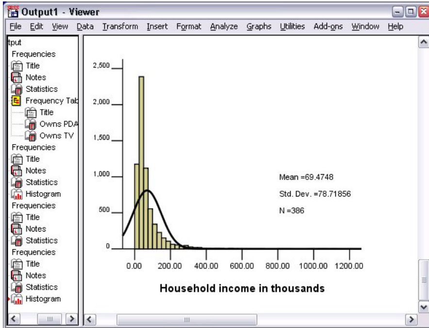
그림 29. 히스토그램
