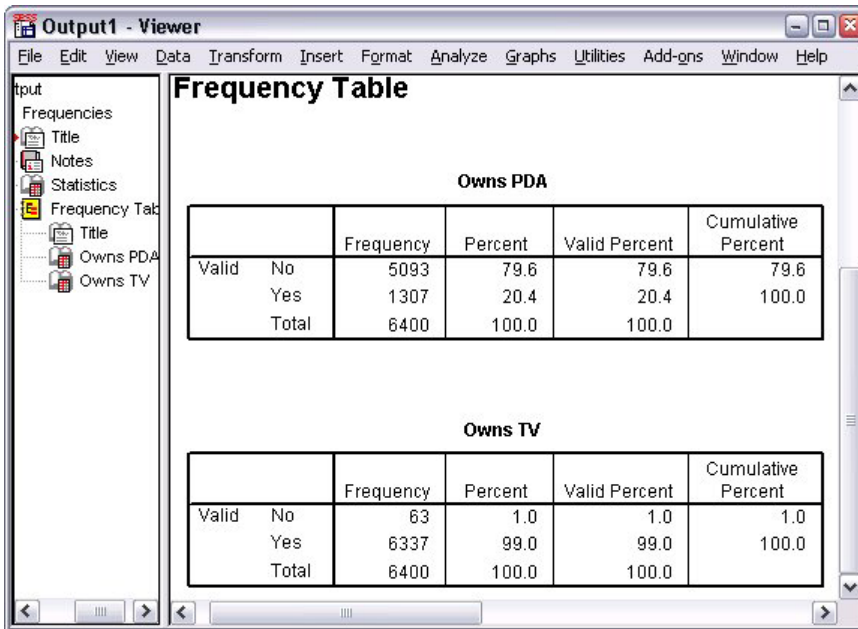
그림 25. 빈도표
