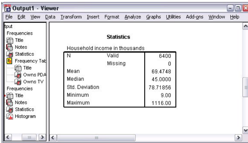
그림 28. 빈도 통계표
