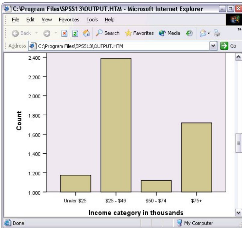
그림 66. HTML에서의 도표
