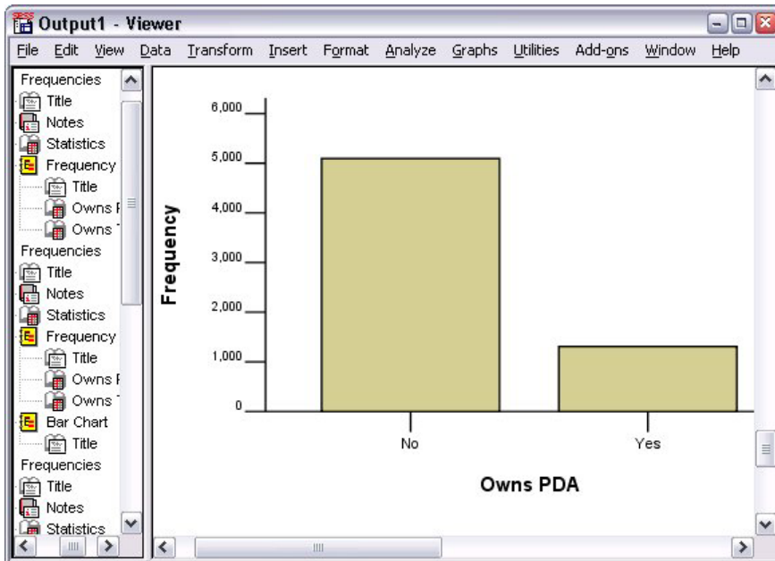
그림 27. 막대도표
