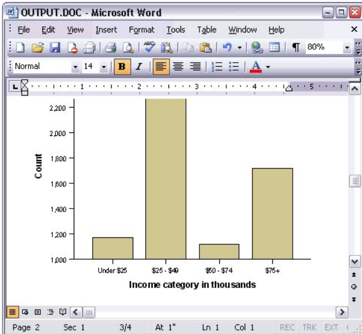
그림 57. Word에서의 도표
