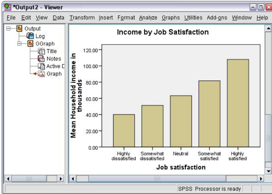
그림 34. 막대도표
