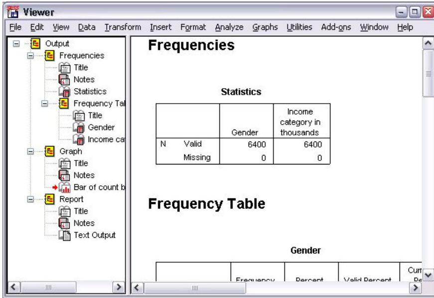
그림 54. 뷰어
