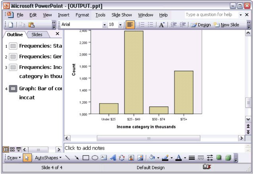
그림 60. PowerPoint에서의 도표
