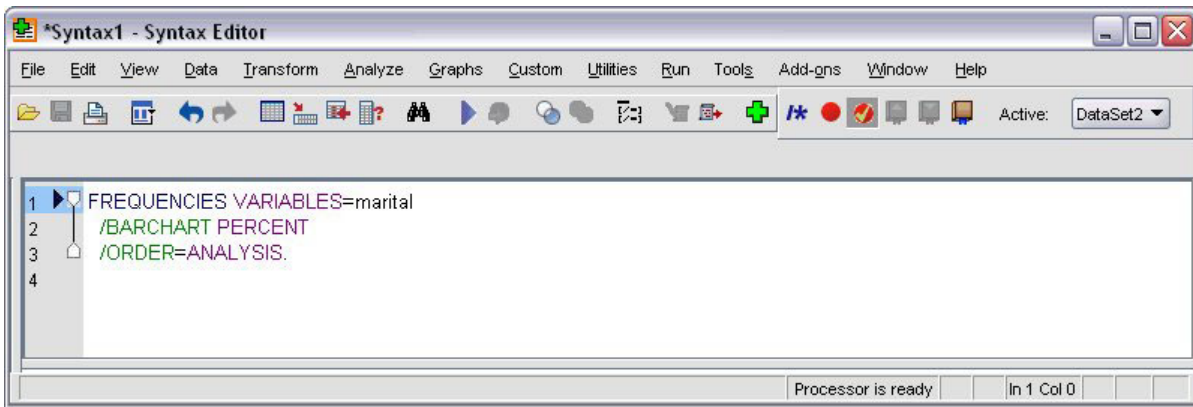
그림 68. 빈도분석 구문
