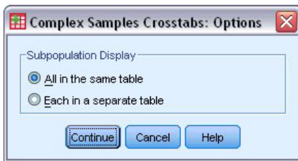
图 5. “选项”对话框
