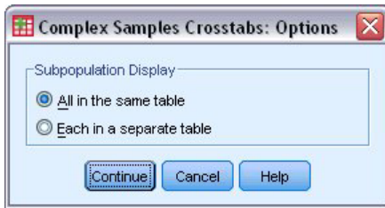
图 8. “选项”对话框
