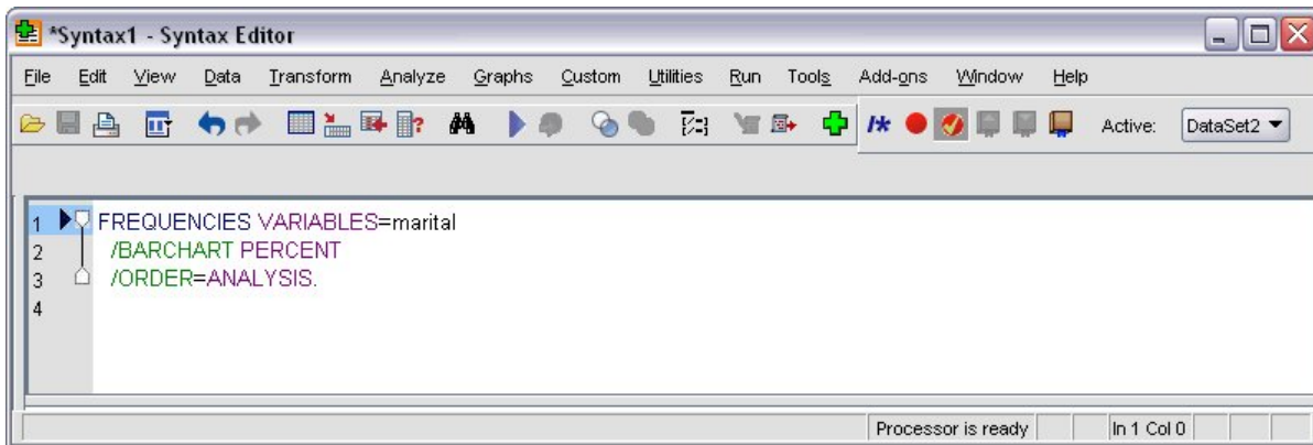
Abbildung 70. Häufigkeitssyntax
