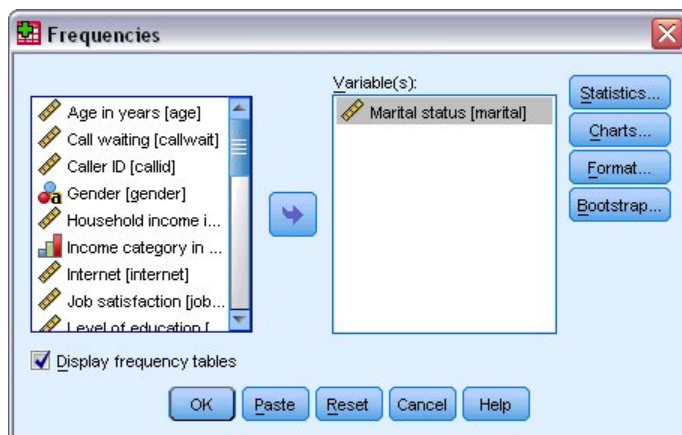
Abbildung 69. Dialogfeld "Häufigkeiten"
