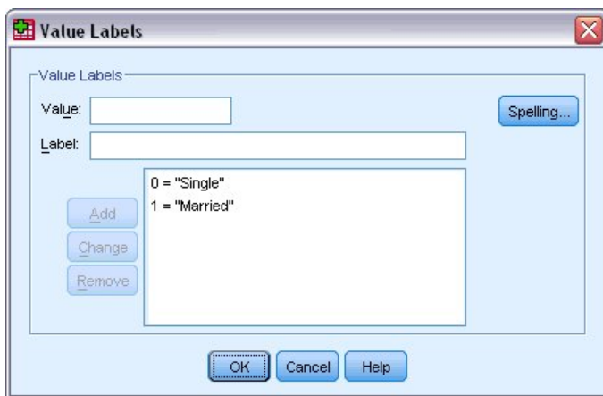
Abbildung 24. Dialogfeld "Wertbeschriftungen"
