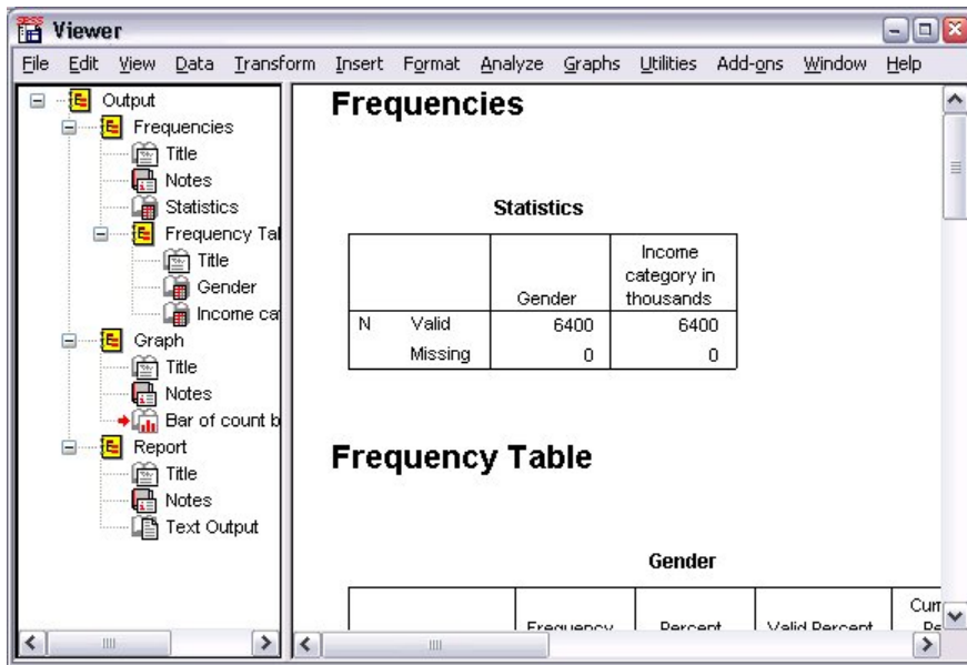
Abbildung 56. Viewer
