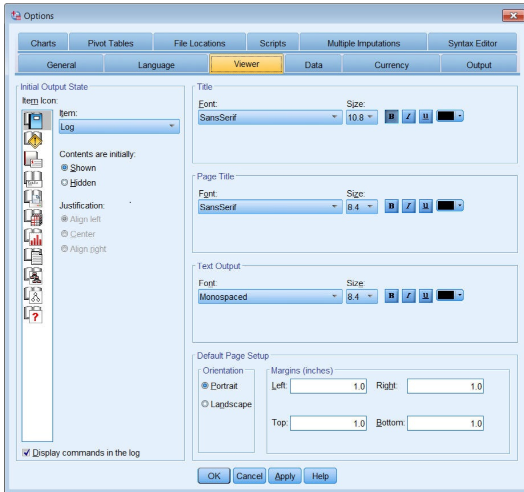
Abbildung 52. Viewer-Optionen
