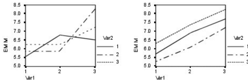
Figura 1. Gráfico no paralelo (izquierda) y gráfico paralelo (derecha)
