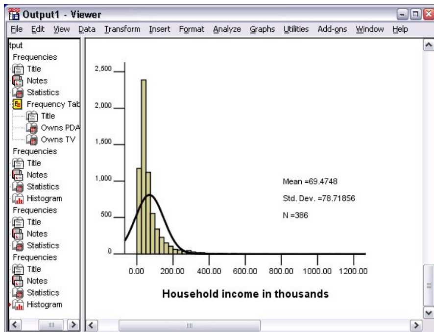
Figura 31. Istogramma
