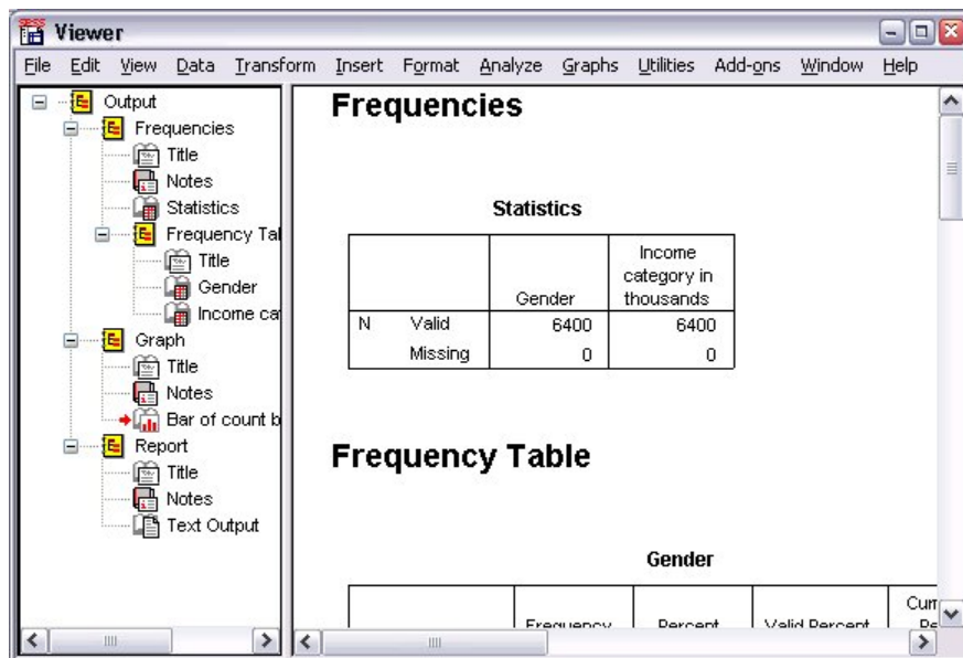
Figura 56. Visualizzatore
