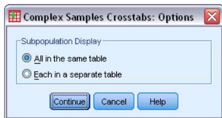
图 4. “选项”对话框
