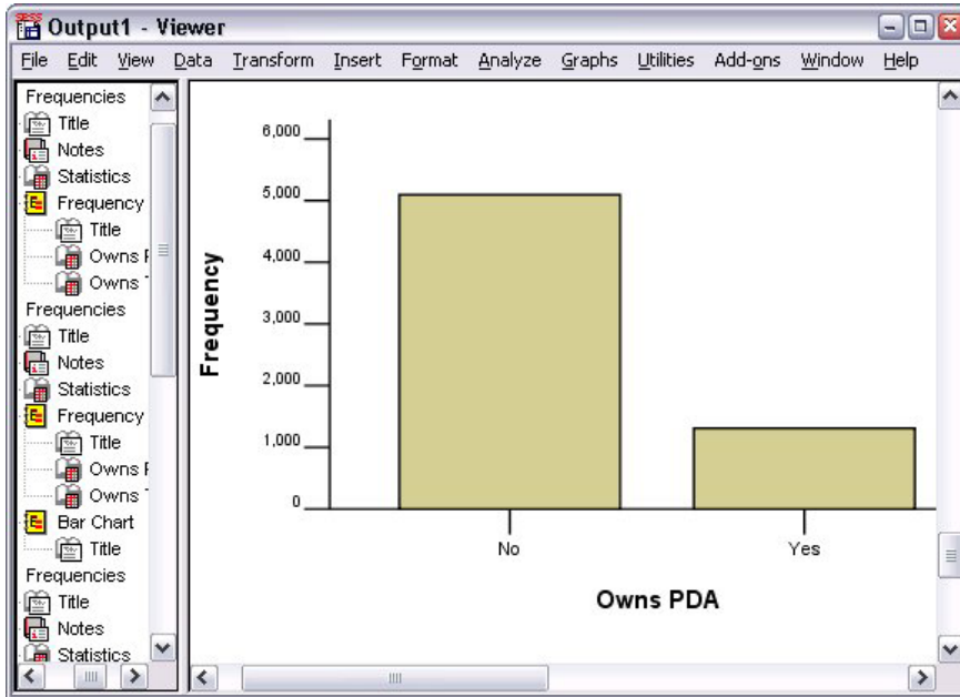
图 29. 条形图
