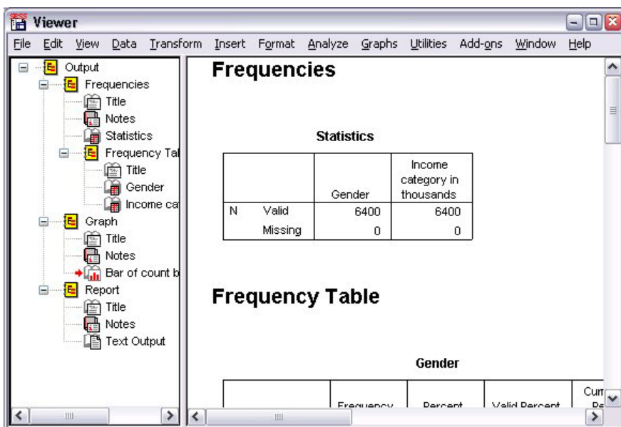
图 56. 查看器(V)
