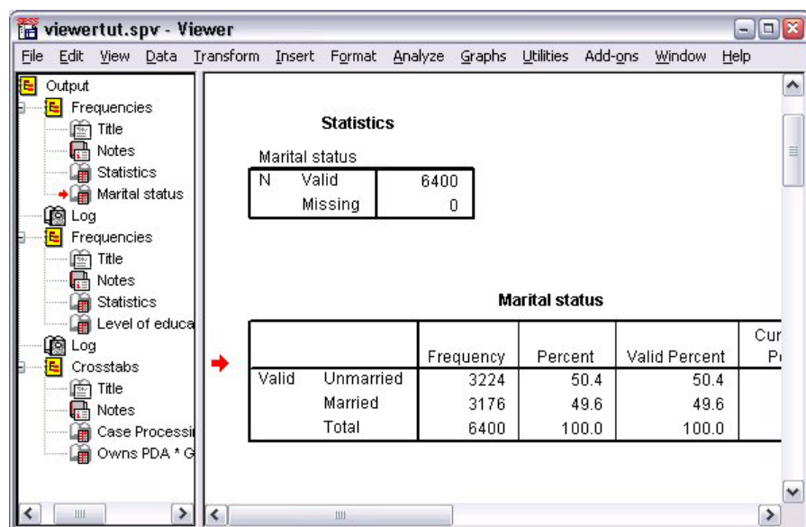
图 37. 查看器(V)
