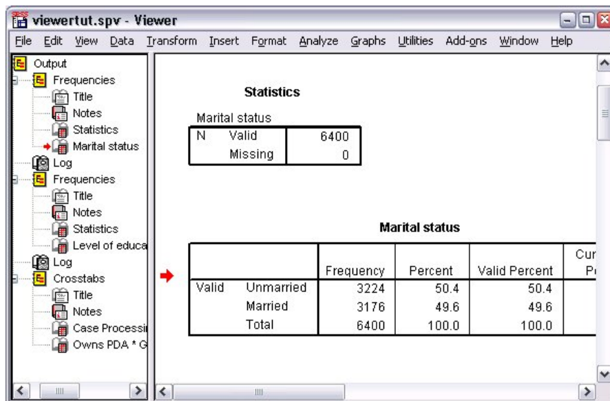
Figure 37. Visualiseur
