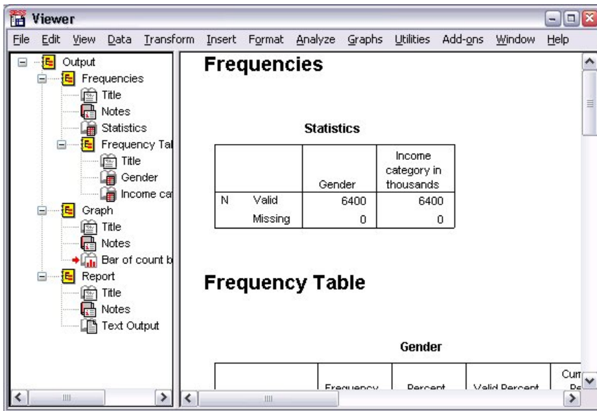
Figure 56. Visualiseur
