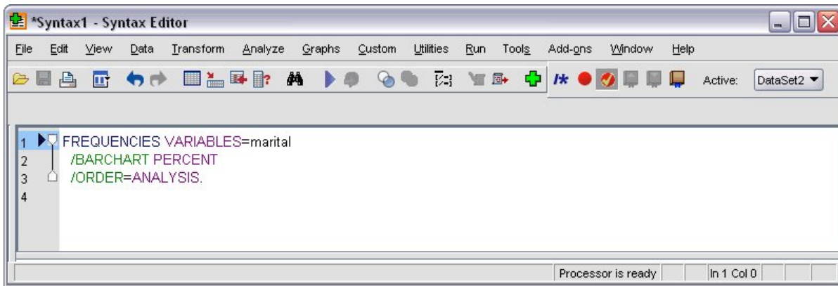
Figure 70. Syntaxe d'effectifs
