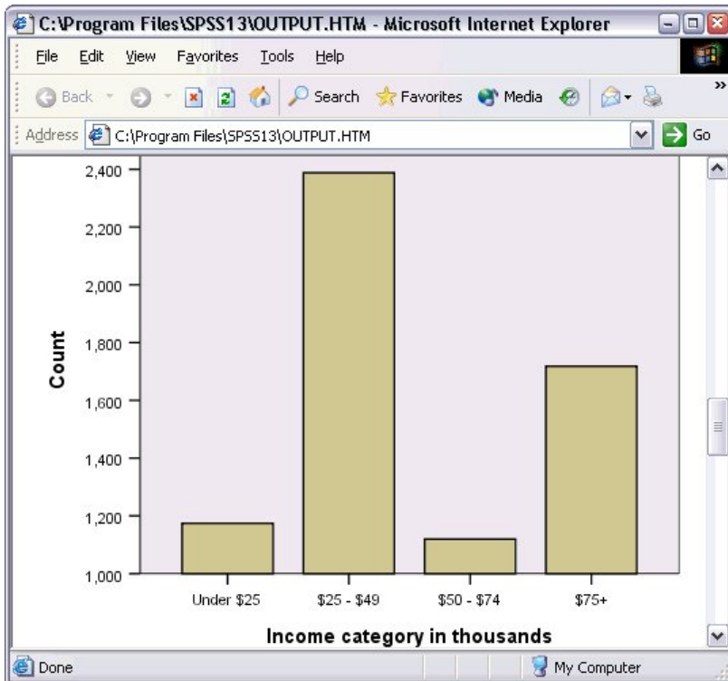
그림 68. HTML에서의 도표
