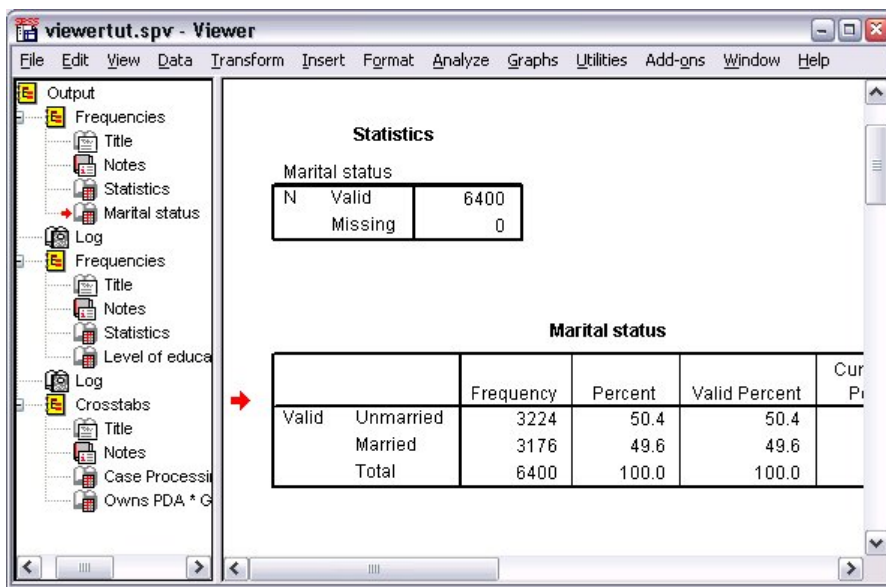
그림 37. 뷰어
