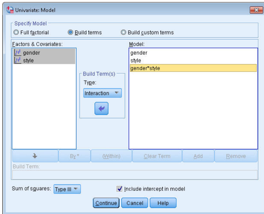
Figura 1. Caixa de diálogo Modelo univariado
