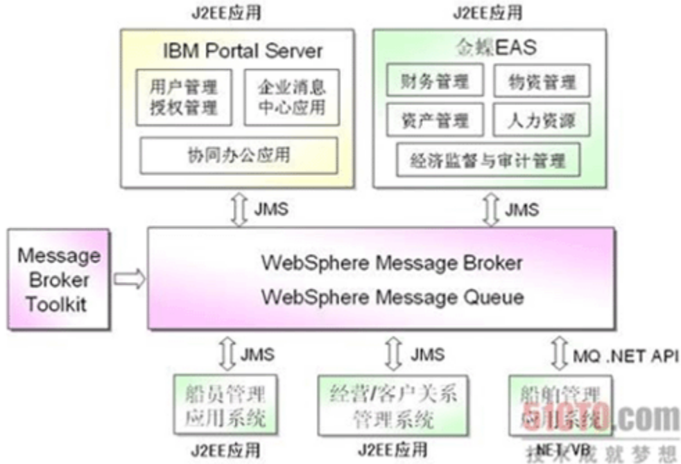
图4：应用系统之间的信息交换
