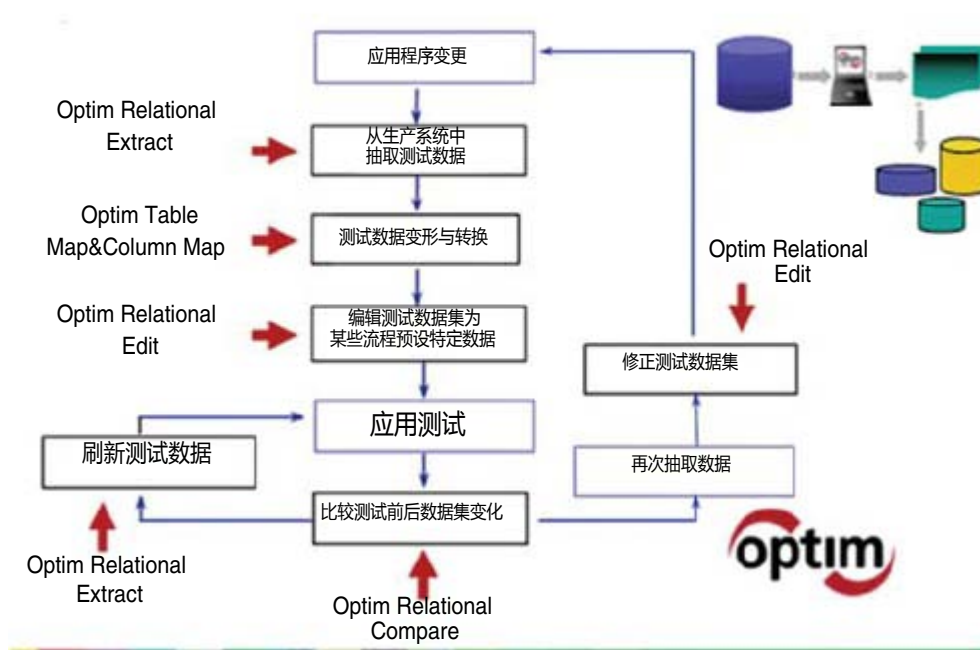
Optim测试数据管理流程
