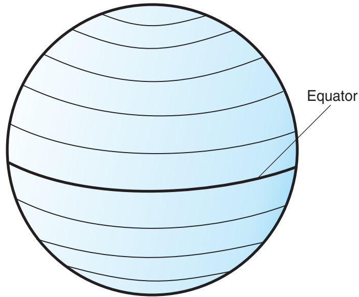
Figure 7. Latitude lines
