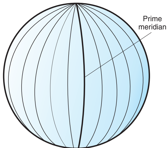
Figure 8. Longitude lines
