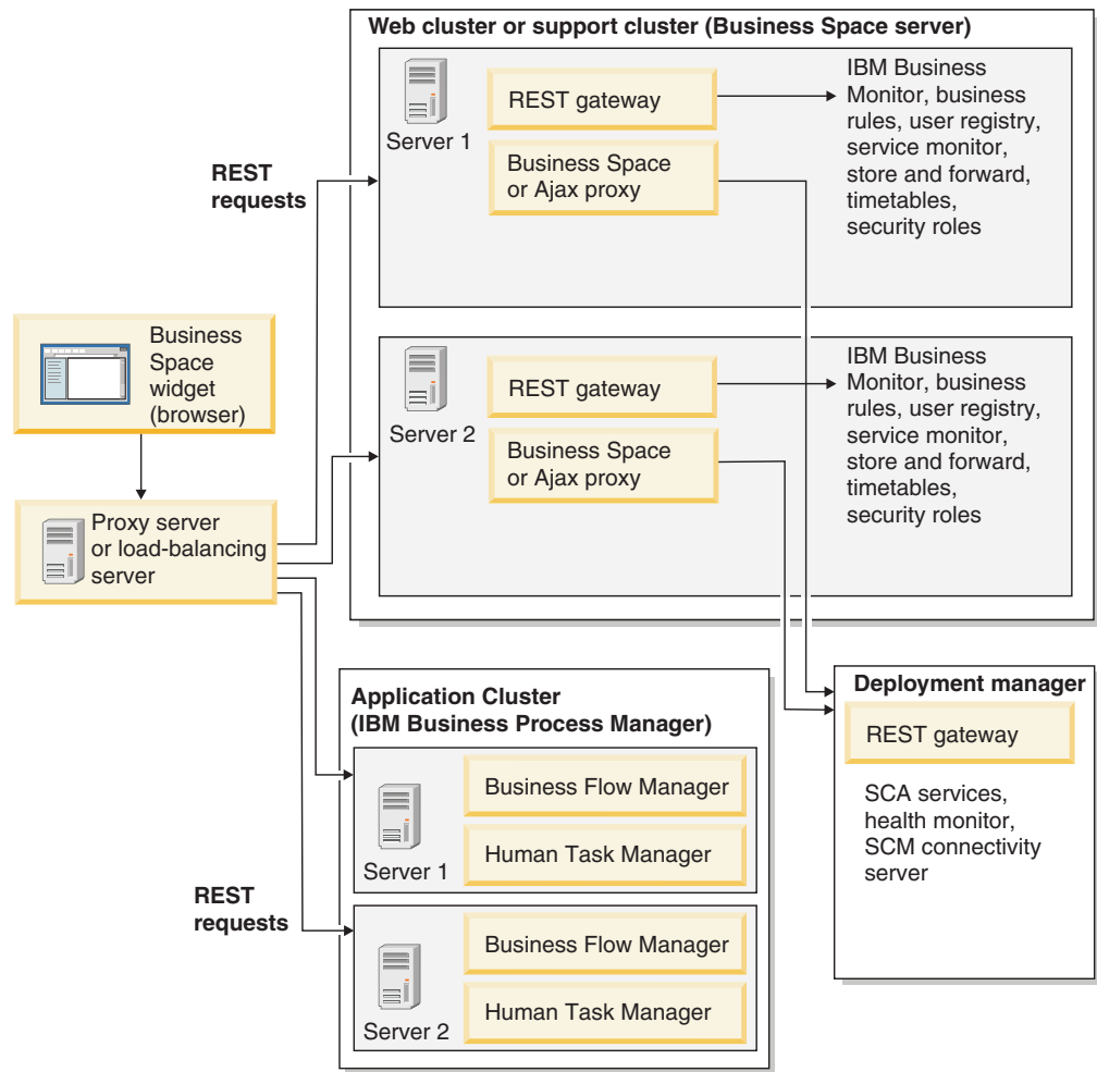
Figura 1. Topologie tipică
