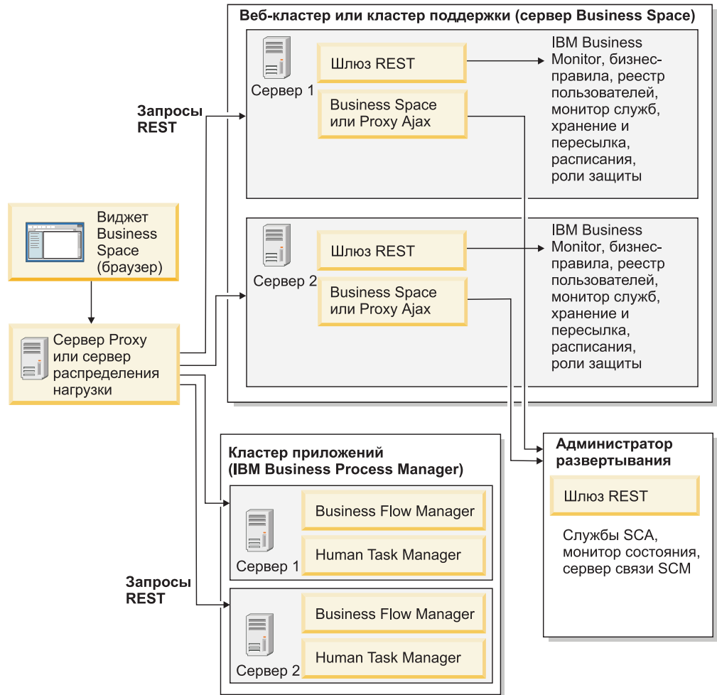
Рисунок 1. Типичная топология
