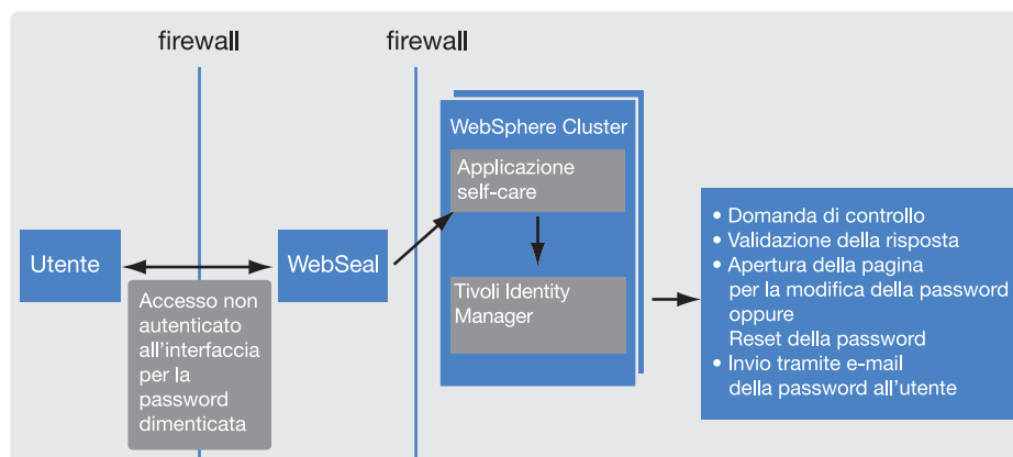
Figura 3.2 Gestione del ripristino e reimpostazione di password dimenticate sfruttando Tivoli Identity Manager e Tivoli Access Manager
