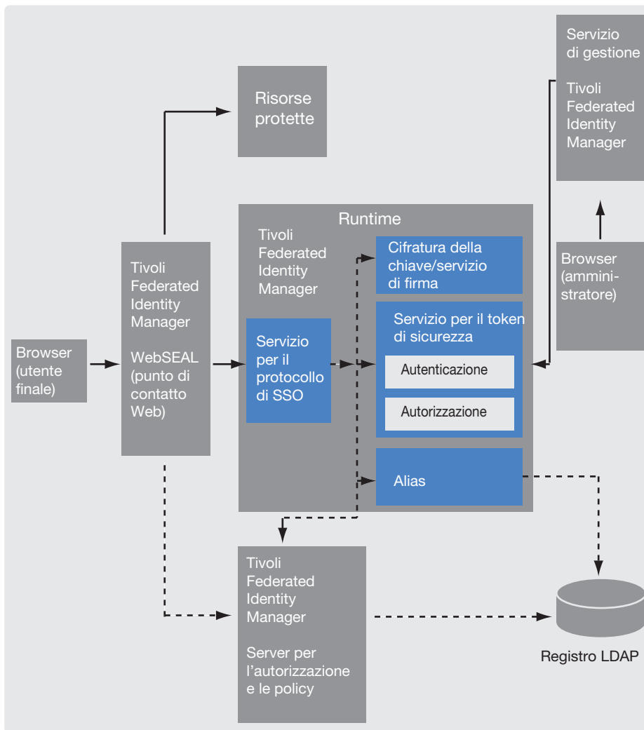
Figura 3.4 Deployment della soluzione Tivoli Federated Identity Manager per il Single Sign-On federato
