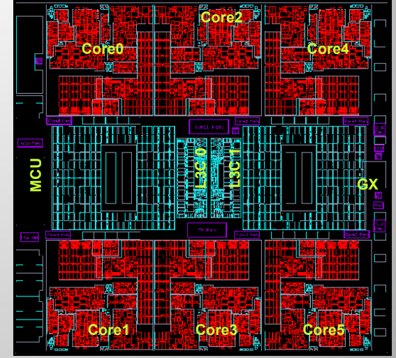
zEC12 PU Yongası: 6 çekirdek, 598 mm 2 vonaa
