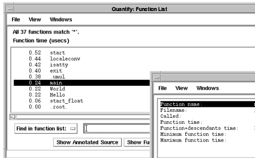
FUNCTION LIST
