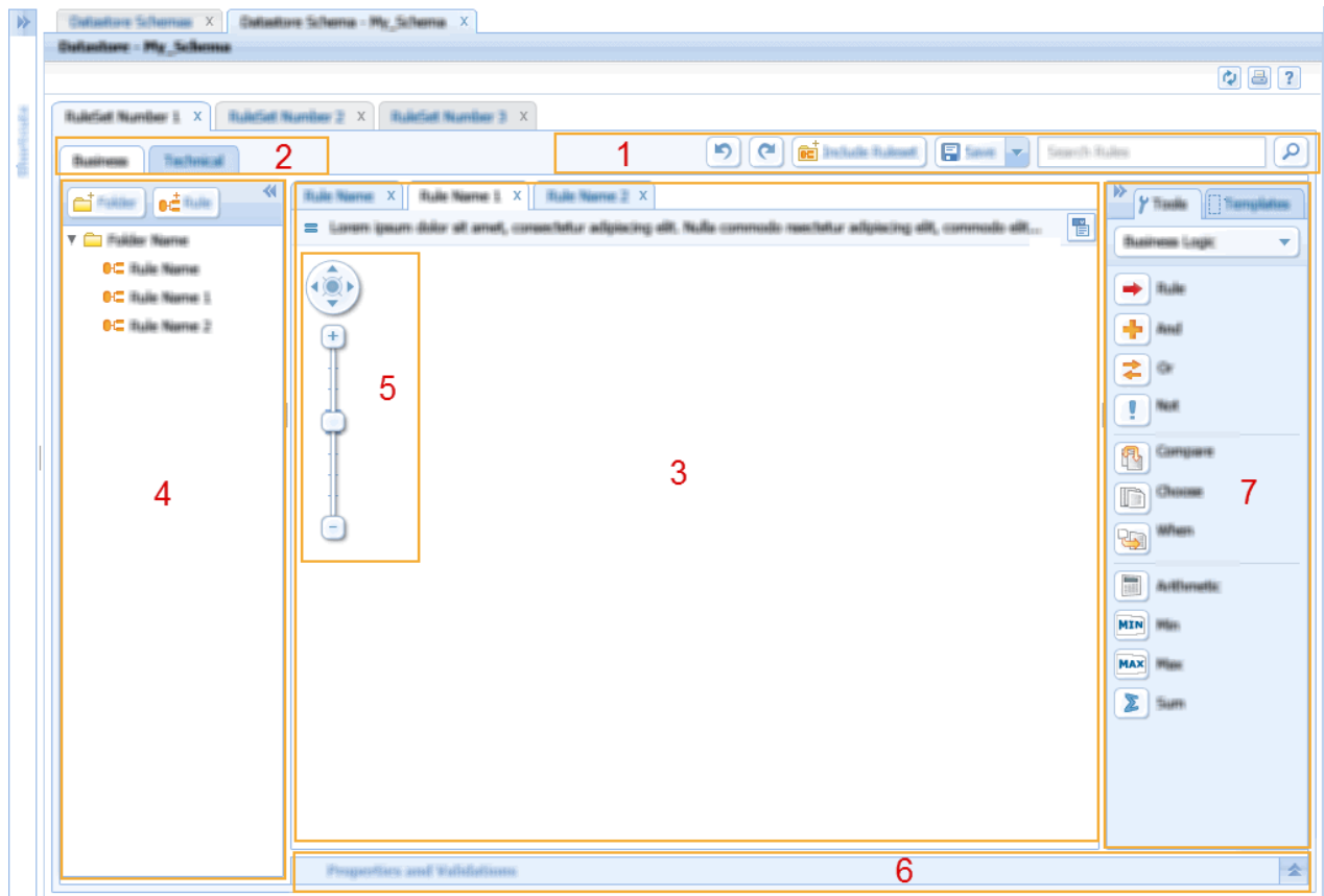
Abbildung 1. CER Editor - Layout
