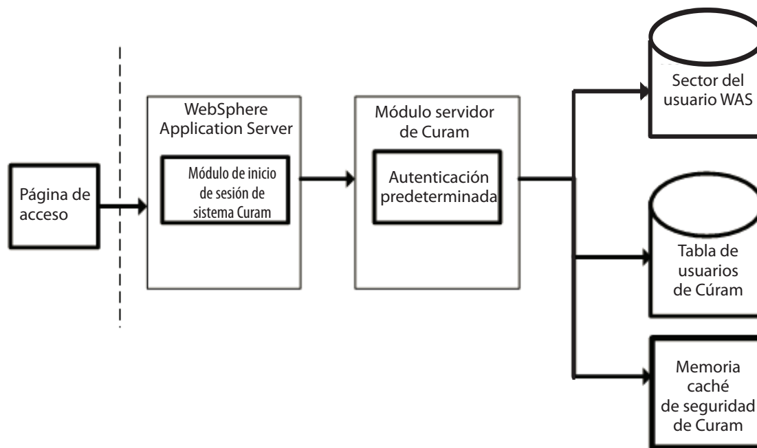
Figura 4. Flujo de autenticación de WebSphere con el registro de usuarios habilitado
