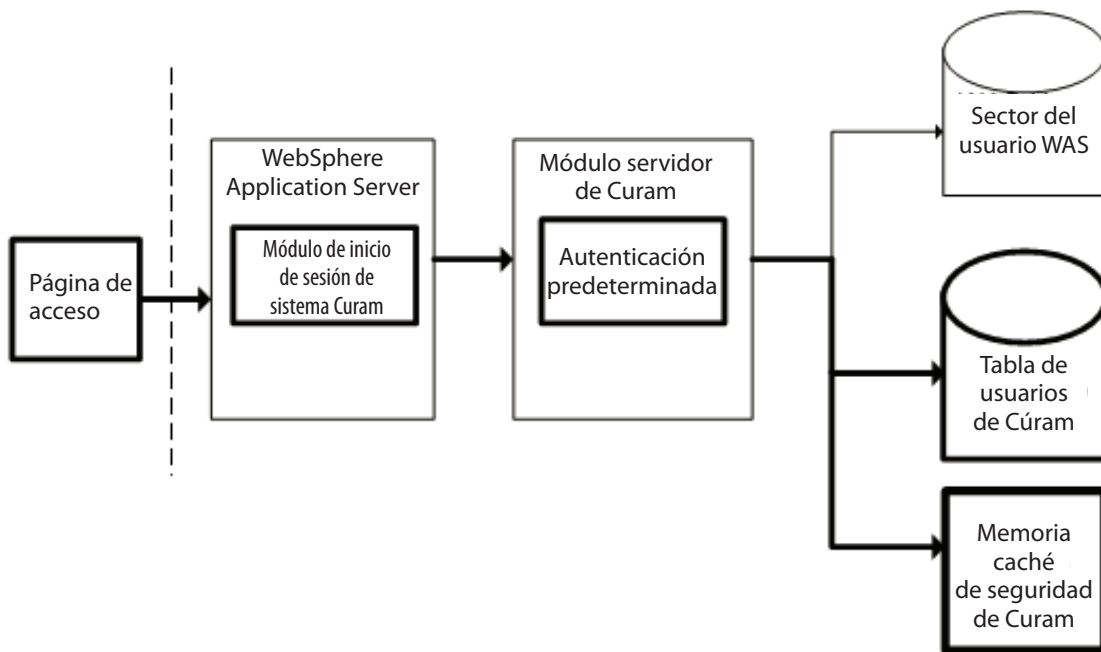
Figura 3. Flujo de autenticación predeterminado de WebSphere
