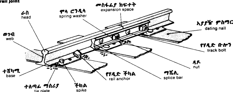
የሃዲድ መጋጠሚያ rail joint
