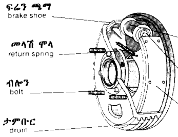
ታምቡር ፍራን drum brake
