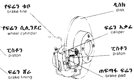
ዲስክ ፍራን disk brake
