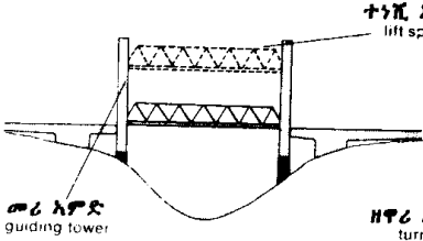
አሳንሮ ድልድይ lift bridge
