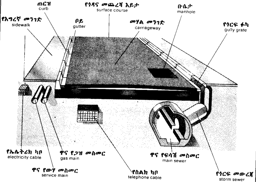
የጎጃና ምስል ክፉይ cross section of a street
