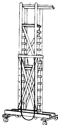
ማማ መሰላላ ladder scaffold
