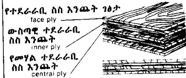
ተሸፋኝ ስስ እንጨት core plywood
