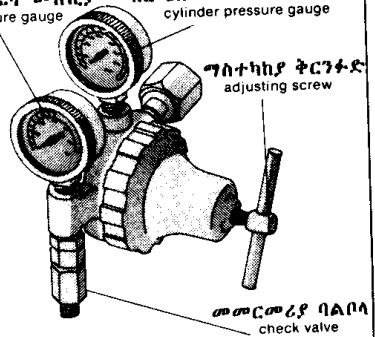
በርሜሎ እየር ግፊት መለኪያ cylinder pressure gauge
