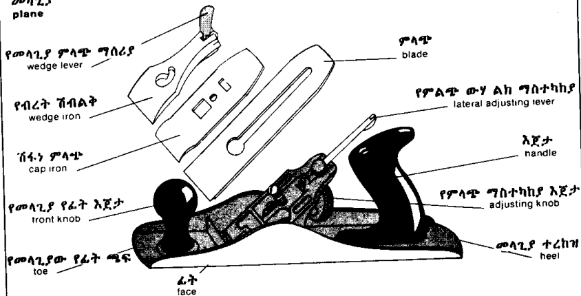
መላጊያ plane
