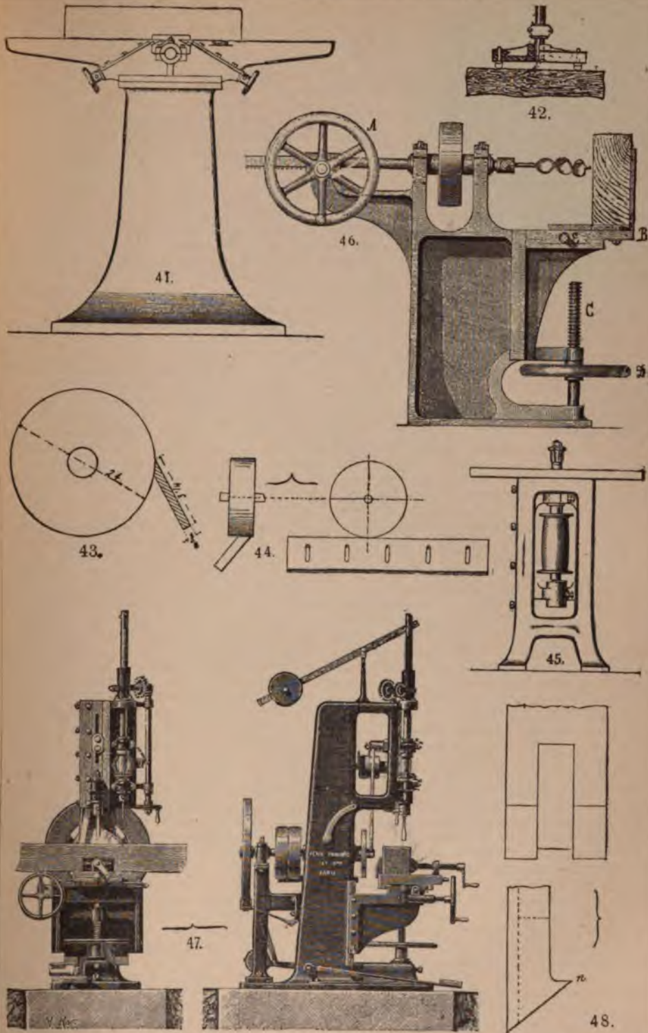
41. Английская универсальная строгательная машина. 42. Рѣжущій аппарат параллельно-строгательнаго станка. 43 и 44. Способы ватачивания ножей тангенциально-строгательныхъ станковъ. 45. Обыкновенный фрезерный станокъ. 46. Горизонтальный сверлильный станокъ. 47. Сверлильно-долбежный станокъ. 48. Устройство долота въ долбежномъ станкѣ.
