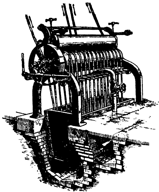
1-వ పటము : బట్టలను నీటిలో బాడించి పిండు యంత్రము
