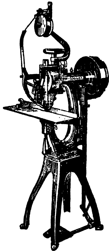
పట్టుయంత్రము
