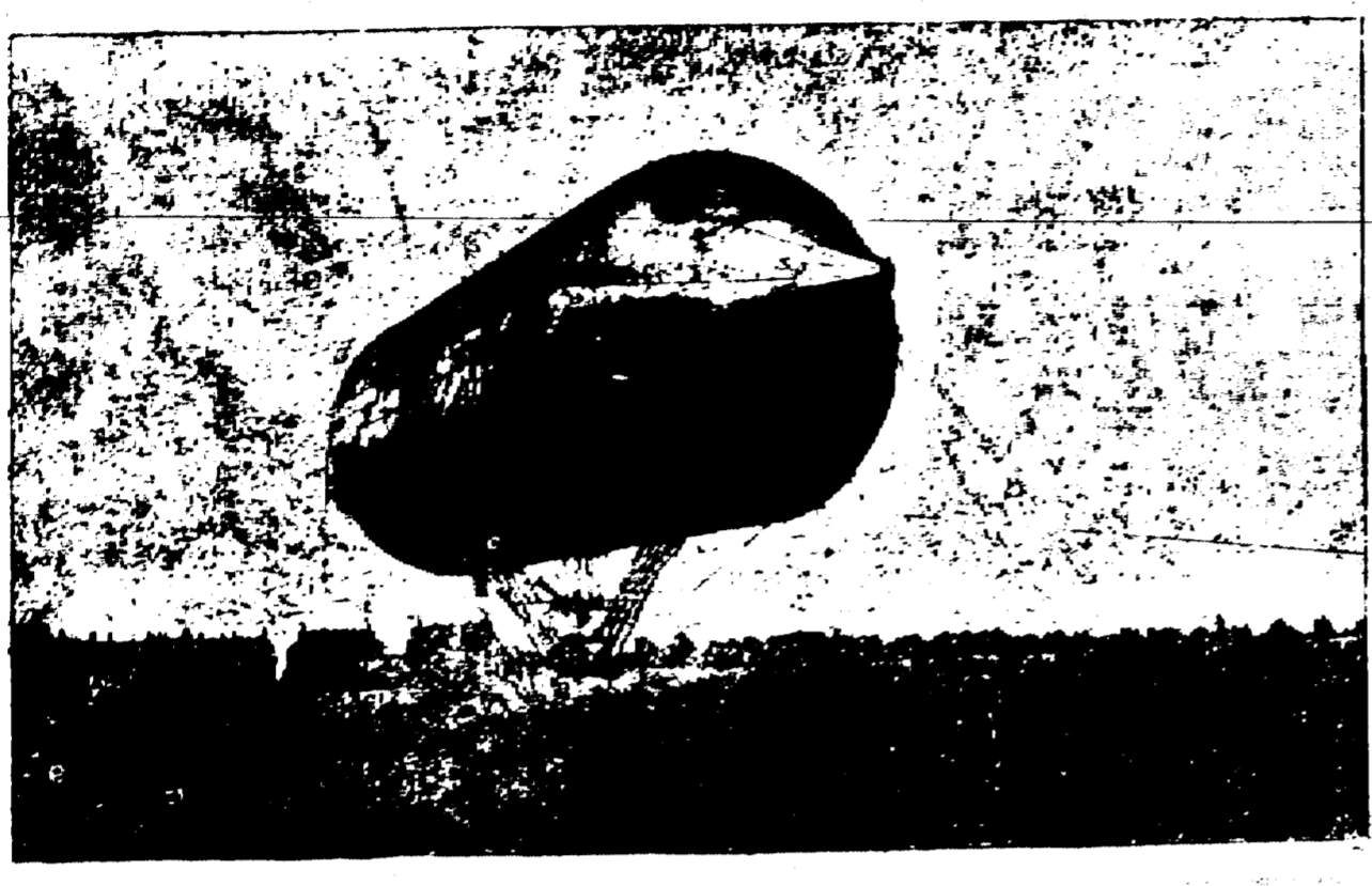
Ballon en aluminium tel qu'on l'a vu aux récents essais d'aérostation à St-Louis.
