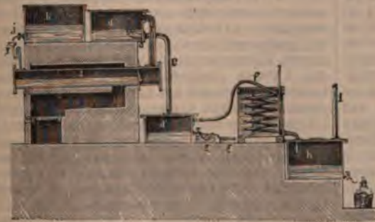
Рис. 13. Приборъ для разложения тяжелого каменноугольного масла дѣйствию высокой температуры.
