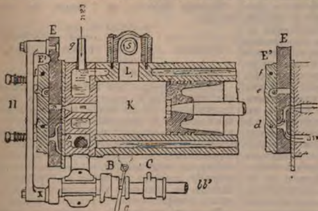
Рис. 5. Золотникъ и поршень Д. Отто.
