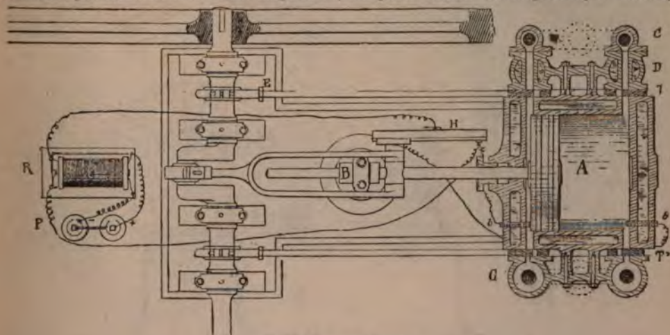
Рис. 1. Двигатель Ленуара.
