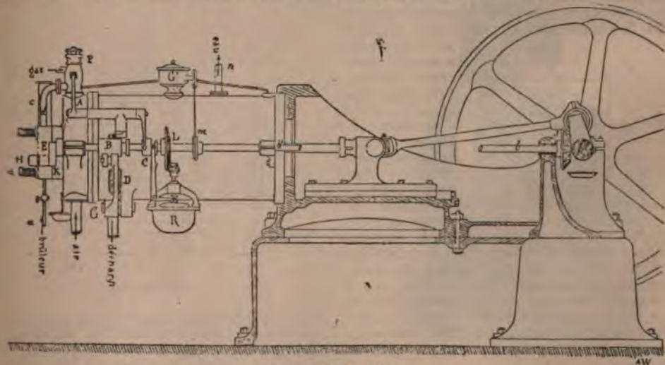
Рис. 2. Двигатель Отто.
