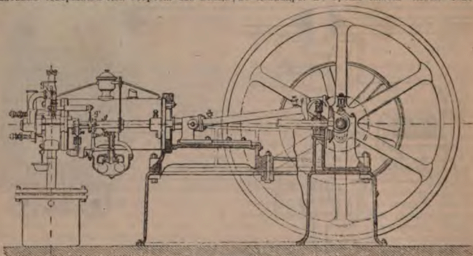
Рис. 3. Двигатель Отто.
