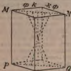
Черт. 1. Схематическое изображение двусос. кристалла; K-O и K'-O' — положение плоскости оптических осей.
