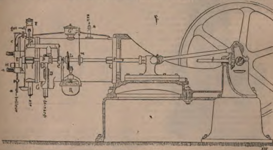
Рис. 2. Двигатель Отто.
