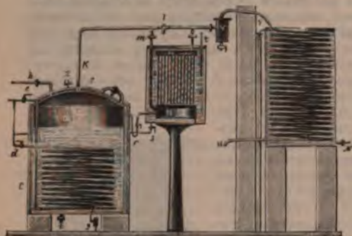
Рис. 9. Дефлегмационный аппарат.
