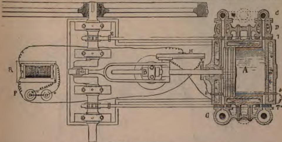
Рис. 1. Двигатель Ленуара.
