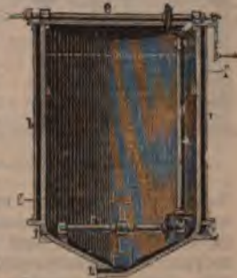
Рис. 8. Мѣшалка для химической обработки продуктовъ перегонки наменпоугольного D .
