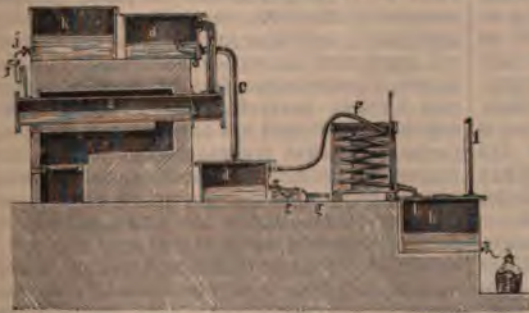
Рис. 13. Приборъ для разложения тяжелого каменноугольнаго масла дѣйствиемъ высокой температуры.
