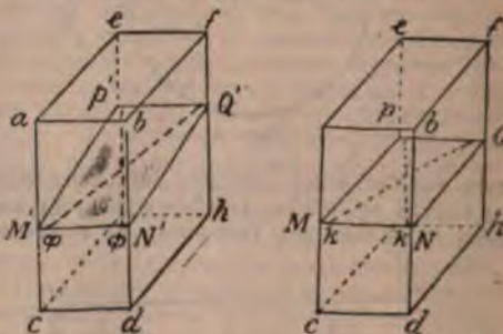
Черт. 11. Ортоклазъ (кварцевый полевой шпатъ). MNP —положеніе плоскости оптическихъ осей для лучей краснаго цвѣта. M'N'P' —положеніе плоскости оптическихъ осей для лучей фиолетоваго цвѣта ( \kappa > \phi ). Плоскость оптическихъ осей вращается при втомъ свое положеніе, поворачиваясь около линіи параллельной ребру кристалла ab .
