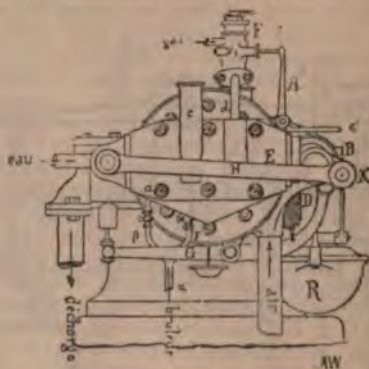
Рис. 4. Двигатель Отто.
