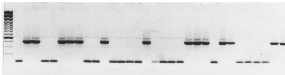
Рис. 4. Электрофорез продуктов RВIP амплификации локуса "SB17—WB17" из генома ячменя в популяции ДН линий Igrі/Triumph. Праймеры из исследуемого локуса: "WB17L": 5'-GTG TCC TCG GAA CGA GCA GG "ISB17L168": 5'-GCC TCA CAG GAT TTT GAG GAG G и праймер с LTR BARE-1: 5'- GGC ATA TTT CCA ACA CCA CTT CC (последовательность LTR выделена полужирным шрифтом). Продукт амплификации 91 основания соответствует наличию ретротранспозиции ретротранспозона BARE-1 в данном локусе, продукт ПЦР в 384 основания — отсутствие ретротранспозиции. Маркер ДНК — "GeneRuler I 100bp DNA Ladder Plus" ("Fermentas") от 100 до 3000 нуклеотидов, "толстая" полоса соответствует 500 нуклеотидам
