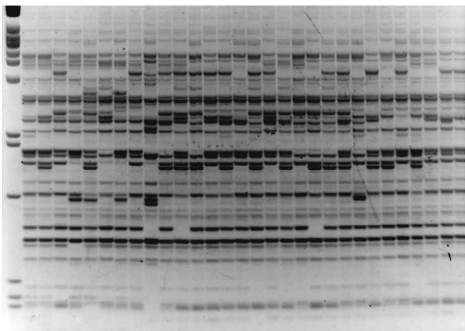
Рис. 3. Электрофорез (в агарозном геле с окрашиванием бромистым этидием) IRAP -амплификации ДНК сортов ячменя с помощью одиночного праймера из LTR-ретротранспозона "Sukkula" (5'-GAT AGC GTC GCA TCT TGG GCG TGA C). Маркер — ДНК фага \lambda , рестрицированная PstI. Условия ПЦР: первая денатурация — 94°C, 2 мин., затем 30 циклов реакции: 94°C — 20с, отжиг 60°C — 20с и элонгация 2 мин, последняя элонгация длится 10 мин. Реакционная смесь на 20 мкл: 50 mM трис-HCl; pH 8,3; 50 mM KCl; 0,01 % Tween-20, 1,5 mM MgCl 2 , 20 нг ДНК, 0,2 мкМ праймера и 1 ед. Taq-полимеразы
