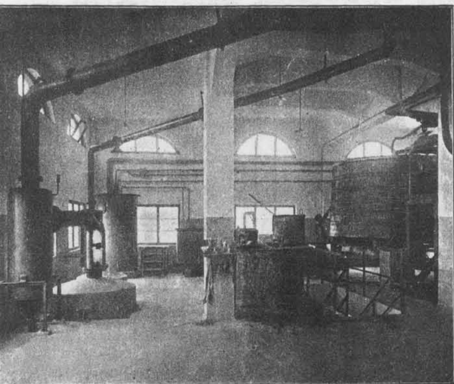
Oddelek za pridobivanje glicerina iz tolšče.
