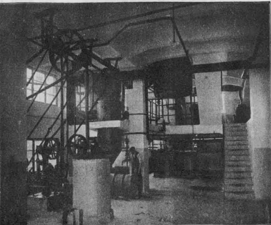
Oddelek za pridobivanje glicerina iz milnega podluga.
