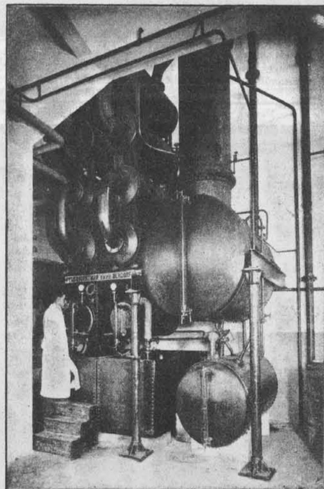
Oddelek za destilacijo glicerina.
