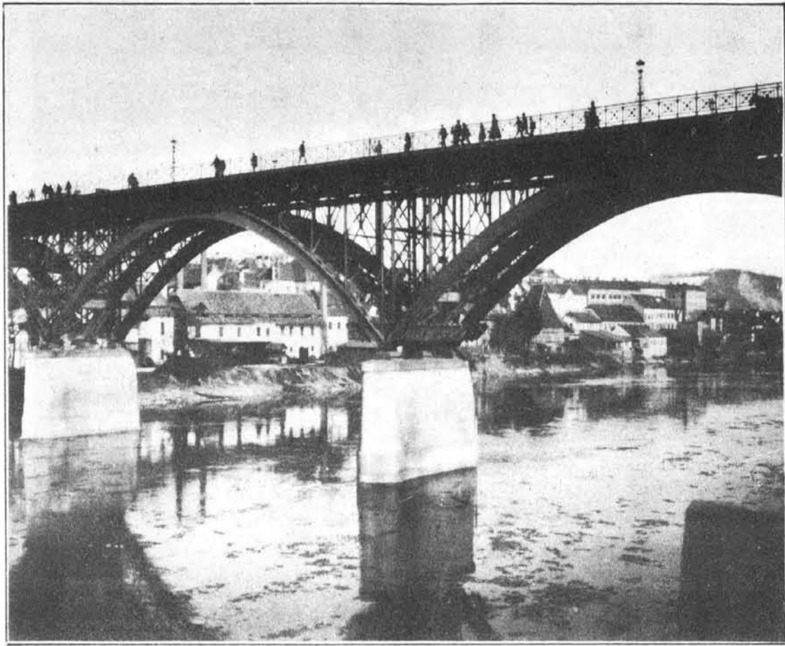
Novi železniški most preko Drave v Mariboru, dolga 122 m, ki je bil dograjen leta 1913.
