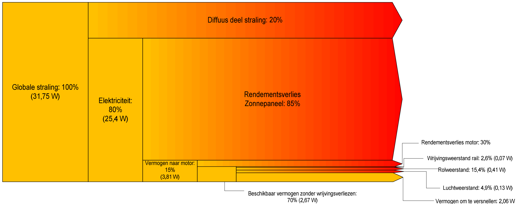
Figuur 7: Energieverliezen op de helft van maximale snelheid (verbeterd)
