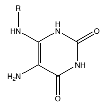
5-amino-6-ribitylamino-2,6-dihydropyrimidinedione
