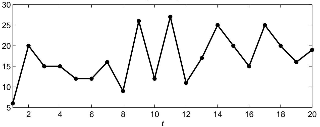
Ungewichteter Gleitender Mittelwert der Breite 3
