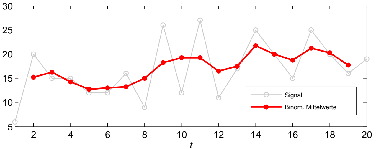
Gleitendes Binomialfilter der Breite 3
